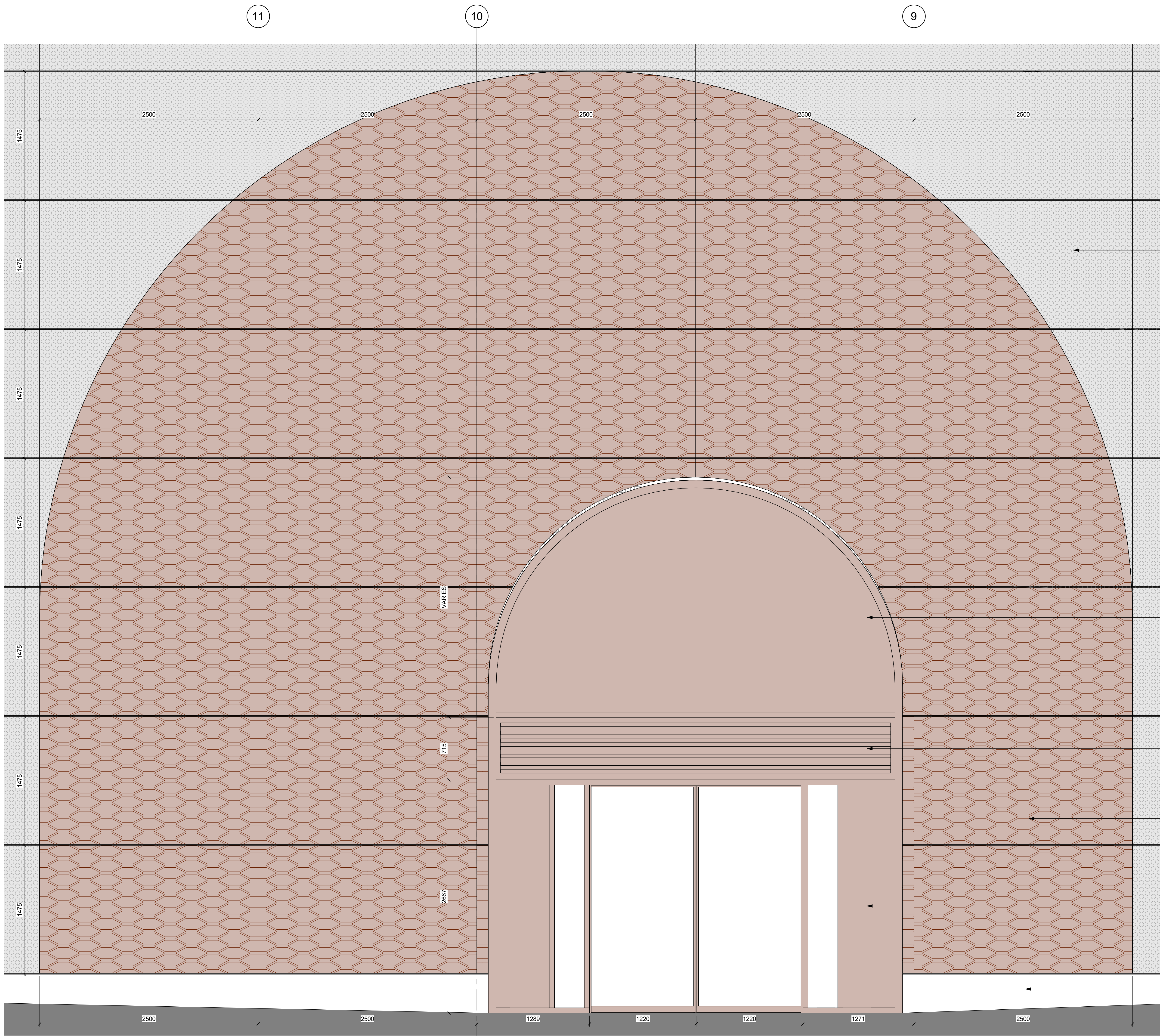
1 Elevation 1 : 20
