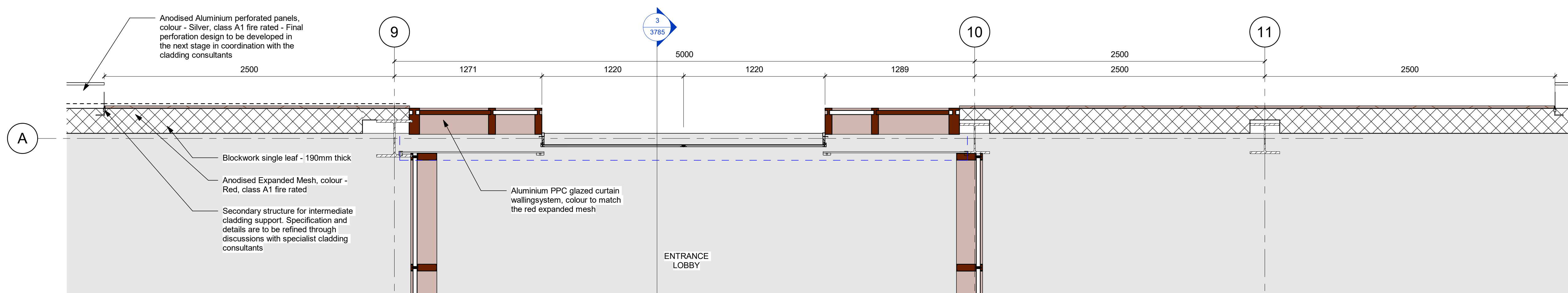
2 Plan 1 : 20
