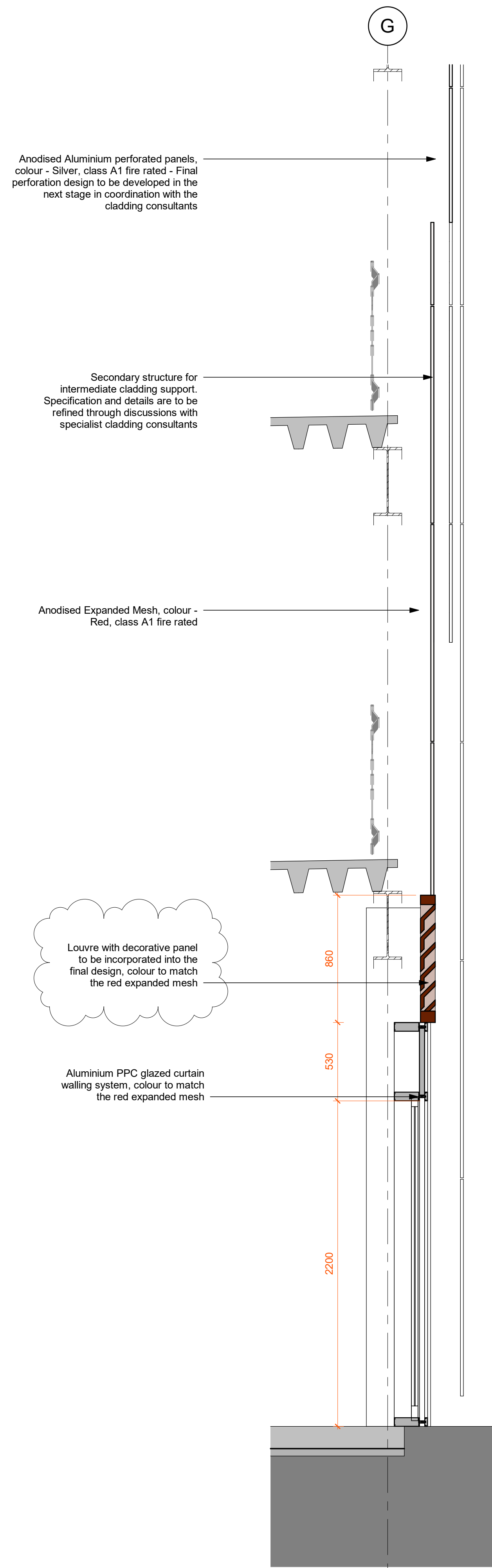
3 Section 1 : 20
