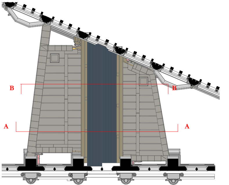
Section Key Plan 1 : 200
