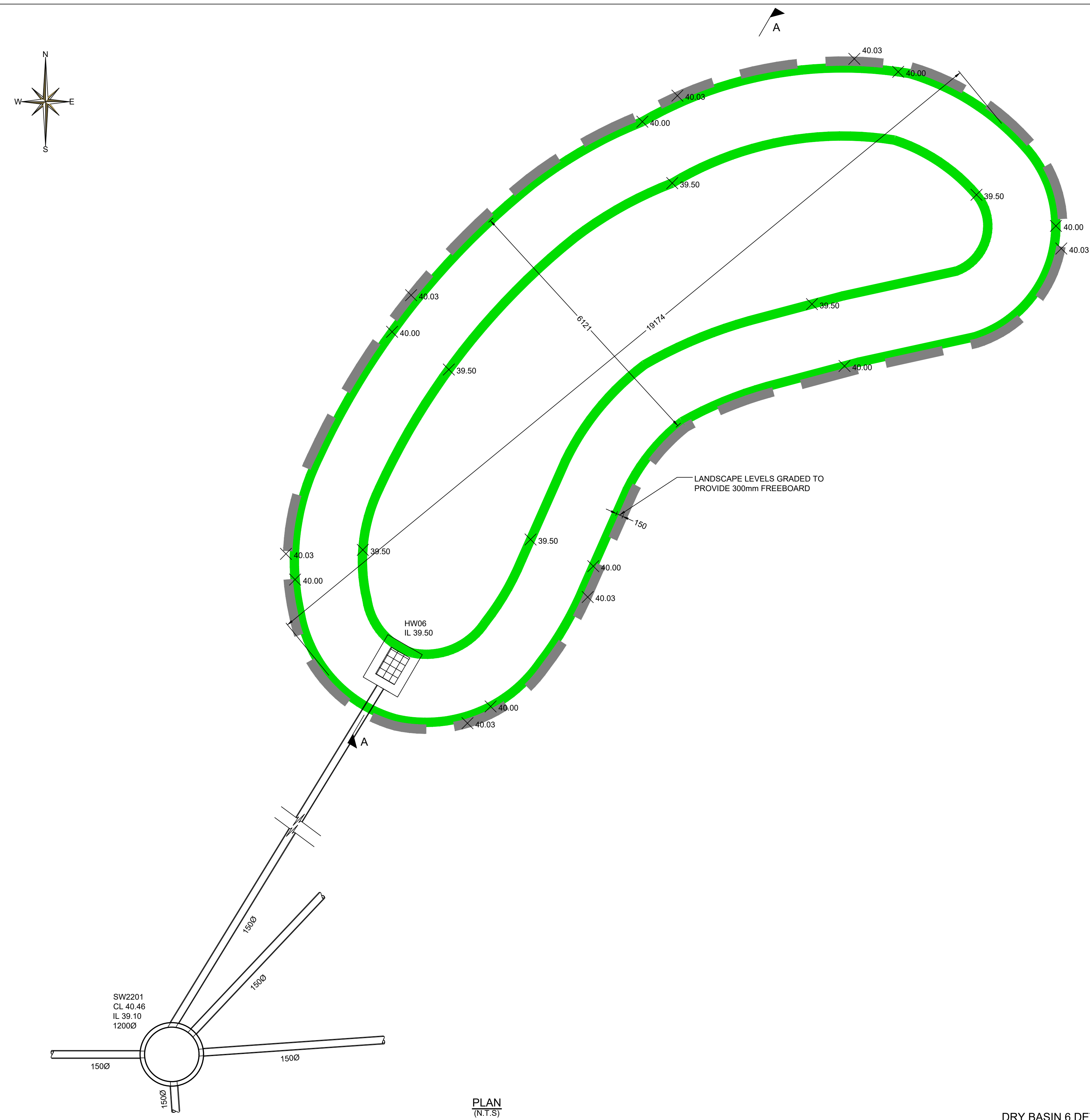
PLAN (N.T.S.) DRY BASIN 6 DETAIL (N.T.S.)
