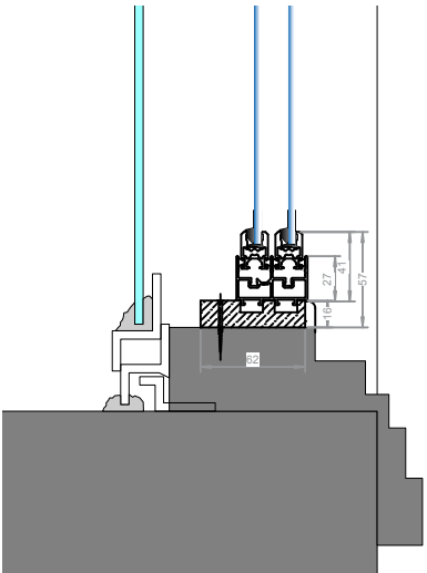
3 Window B Section Scale: 1:5
