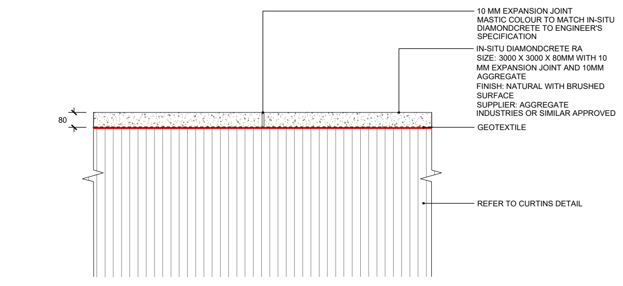
01A 00600 IN-SITU DIAMONDCRETE RA SECTION
