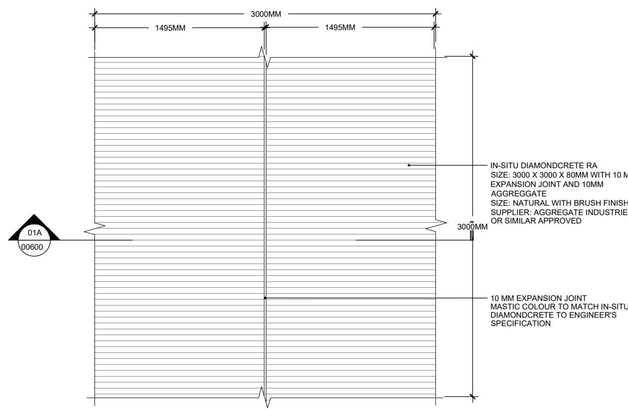
01B 00600 IN-SITU DIAMONDCRETE RA PLAN
