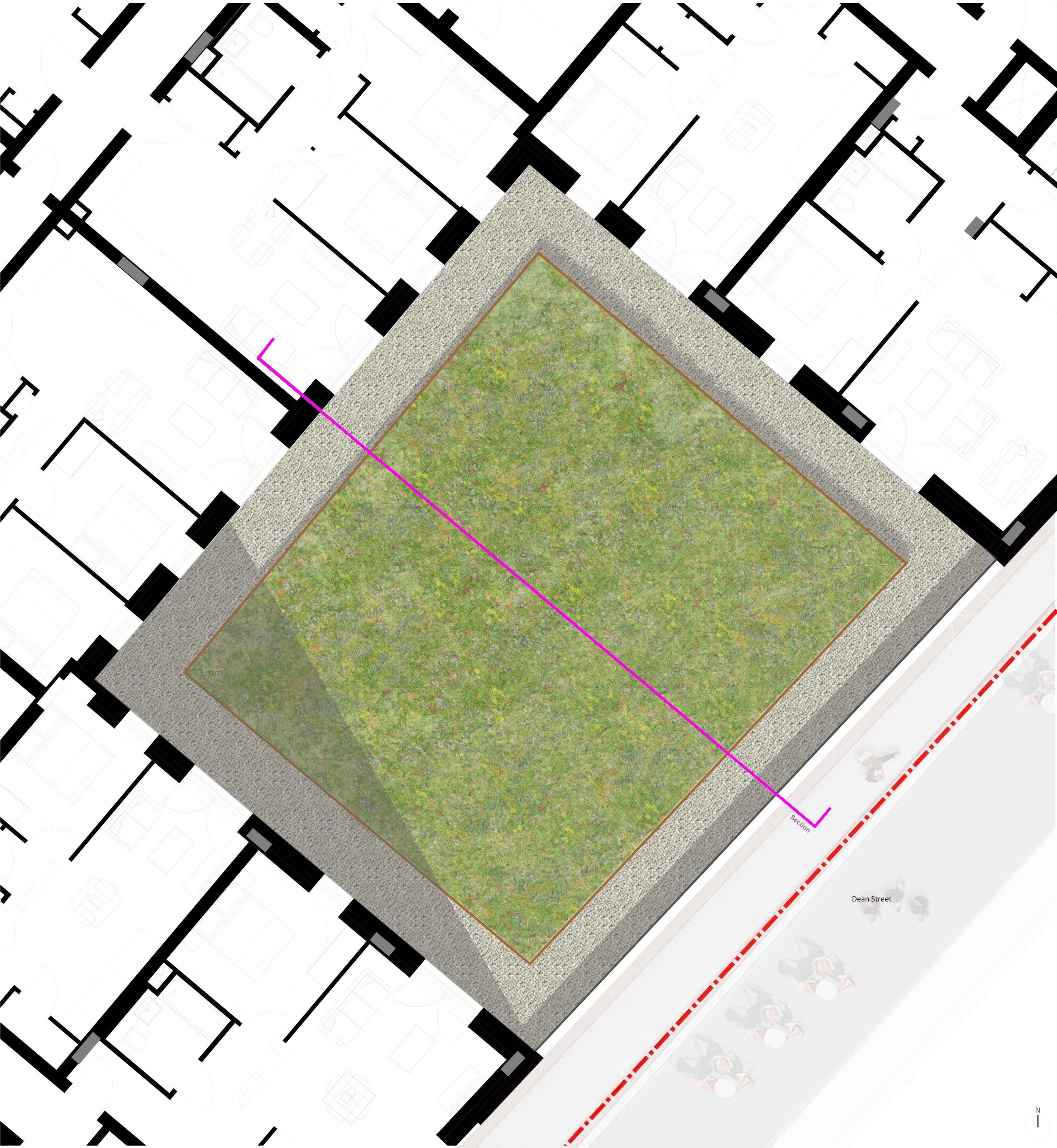
9004 Level 1 Podium Plan 1:50
