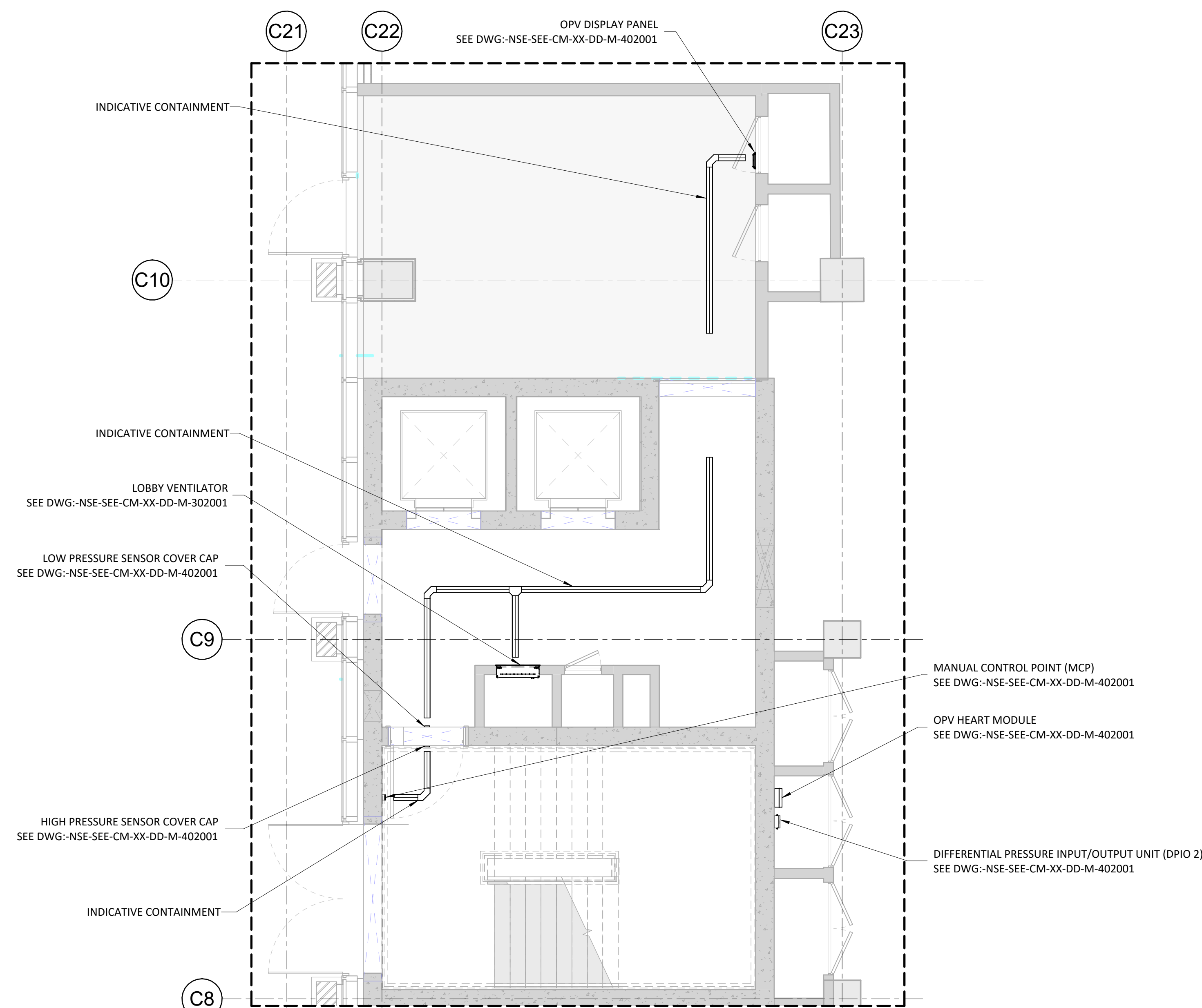
2 DETAIL - STAIR 3 1 : 50
