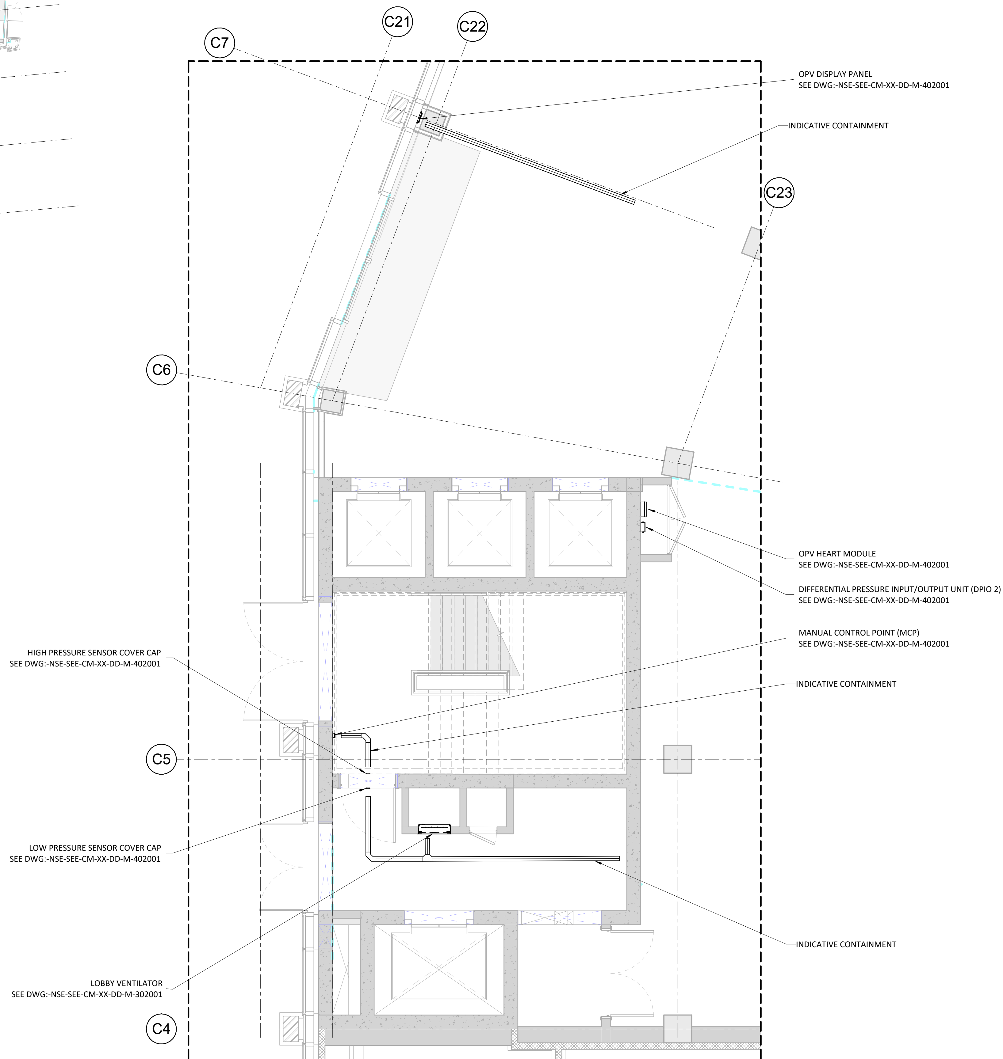
1 DETAIL - STAIR 1 1 : 50
