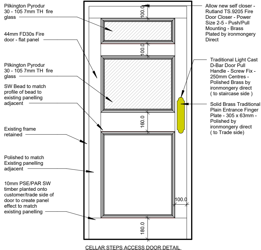
Cellar Steps Access Door 1 : 20
