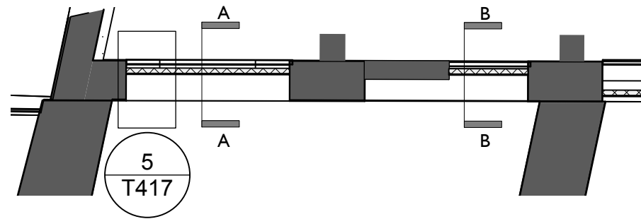
3 LG 1A Plan Scale: 1:100
