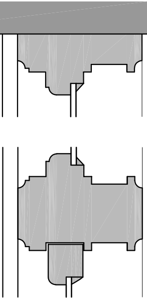
Detail Jamb Plan 1/5
