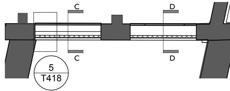
3 LG 1B Plan Scale: 1:100
