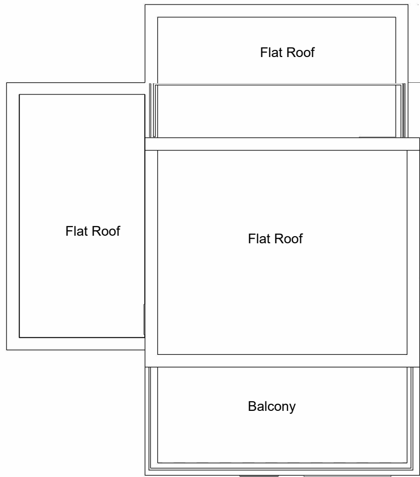
Roof Plan 1 : 100
