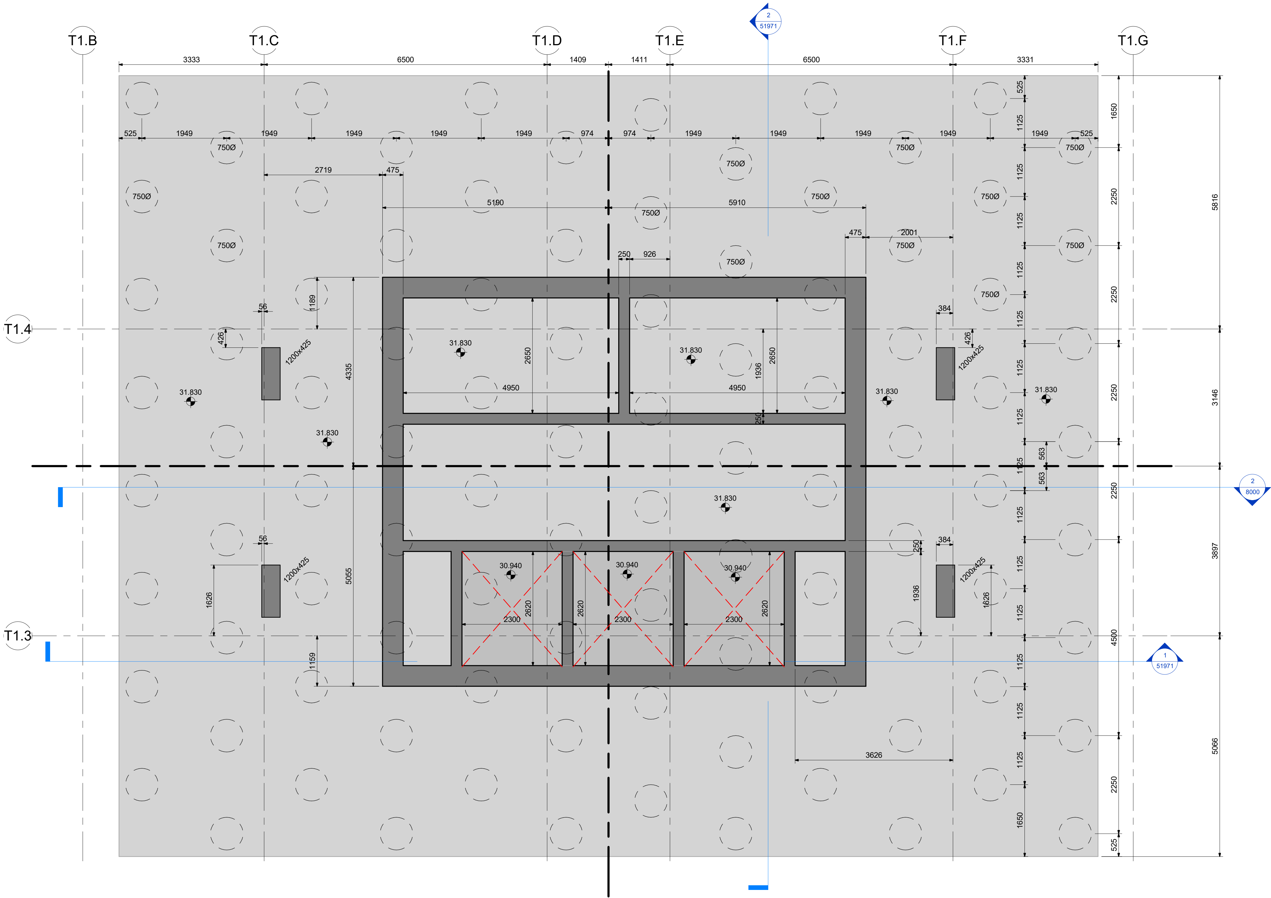
1 CORE BASE G.A 1 : 50
