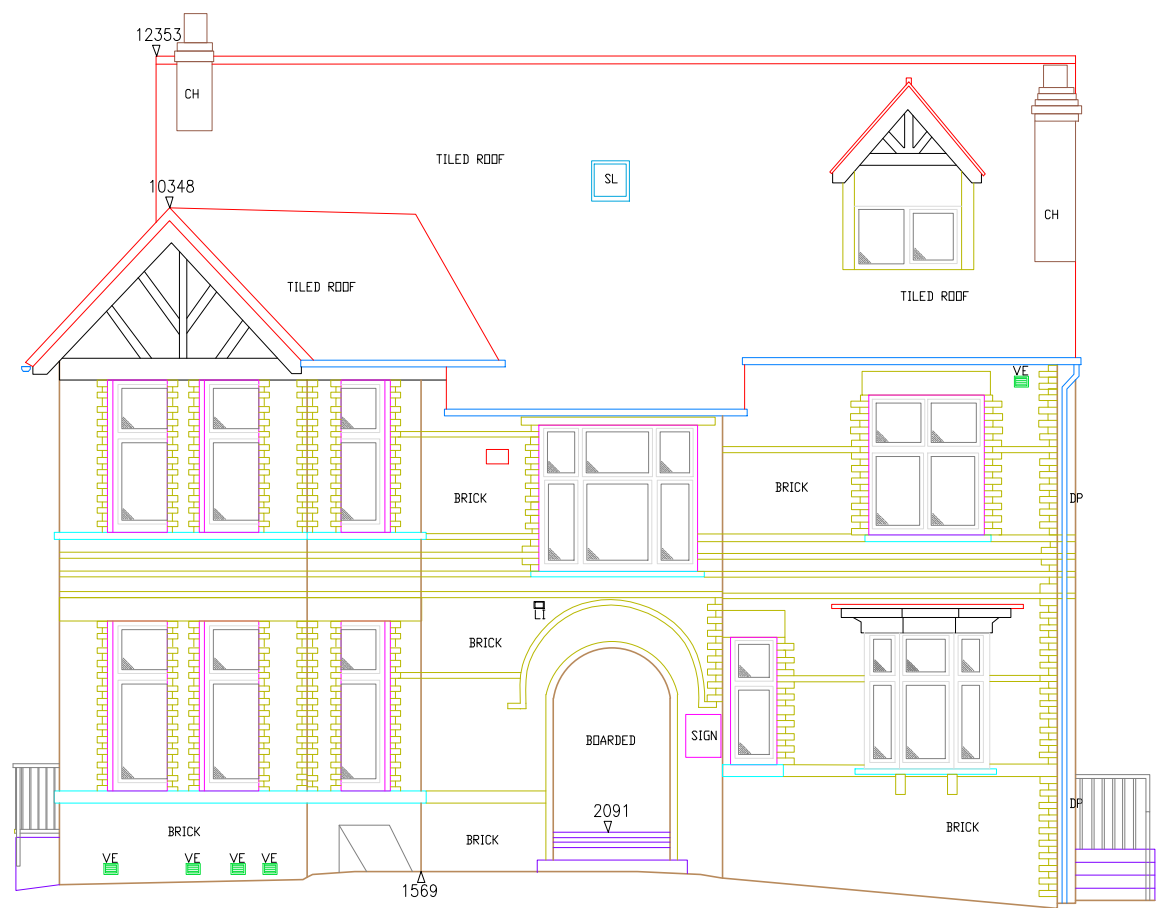
Datum OM NORTH ELEVATION
