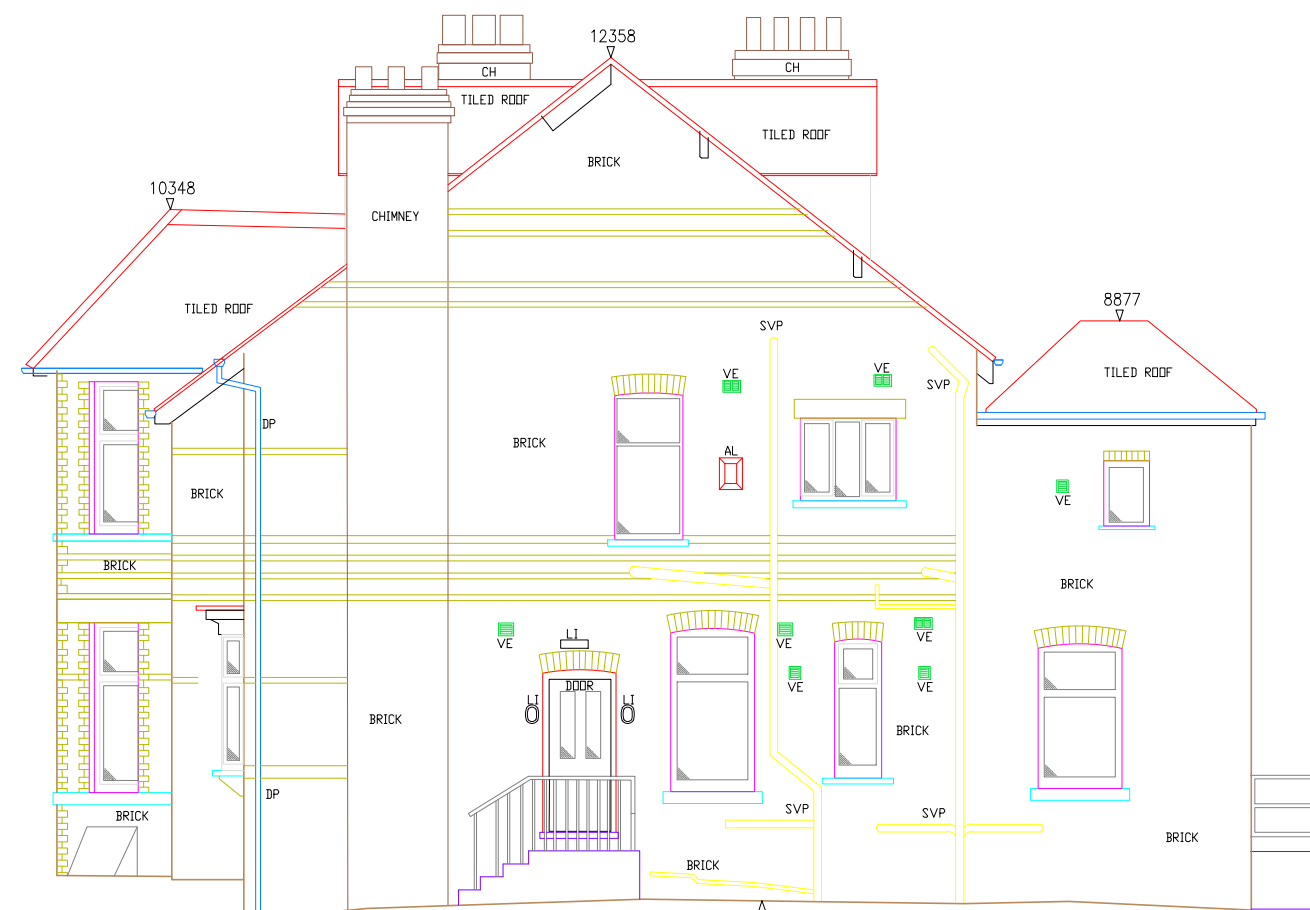
Datum OM WEST ELEVATION
