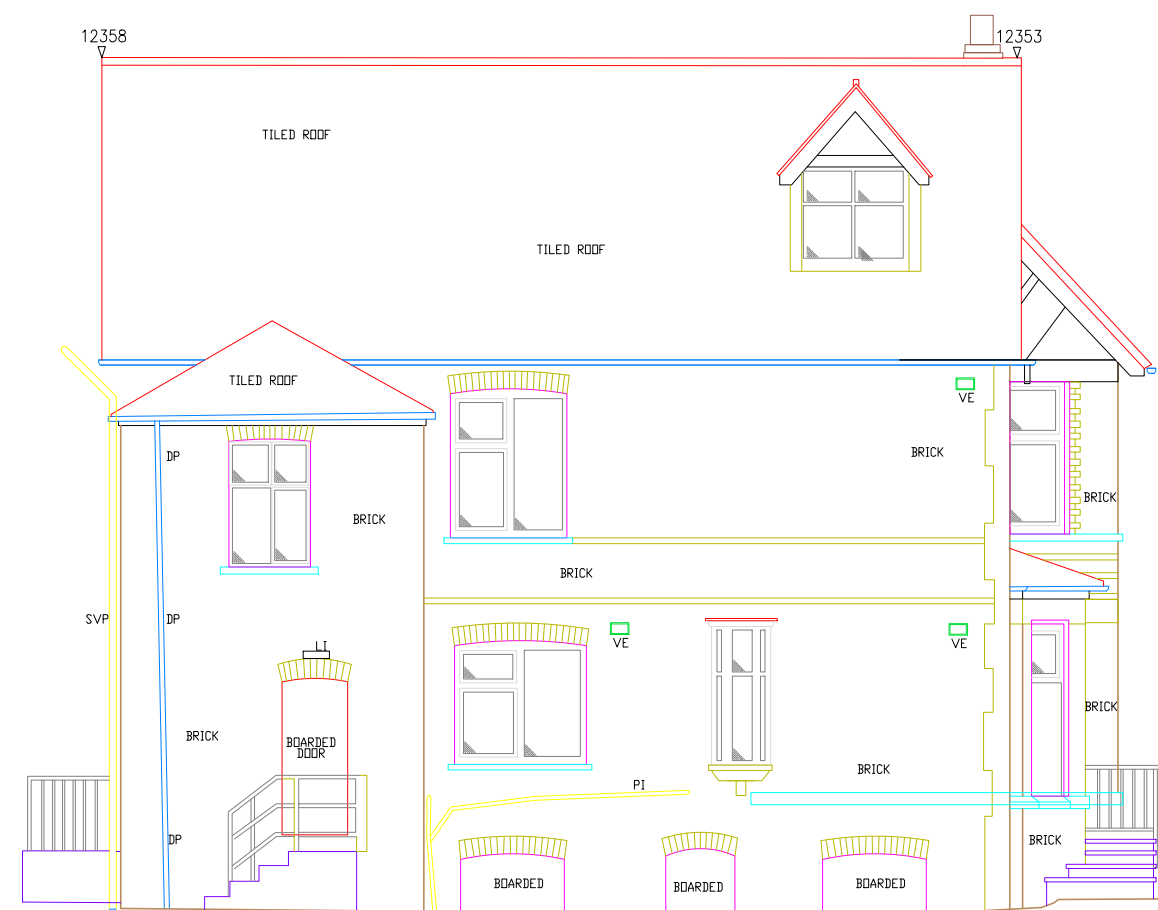
Datum OM SOUTH ELEVATION
