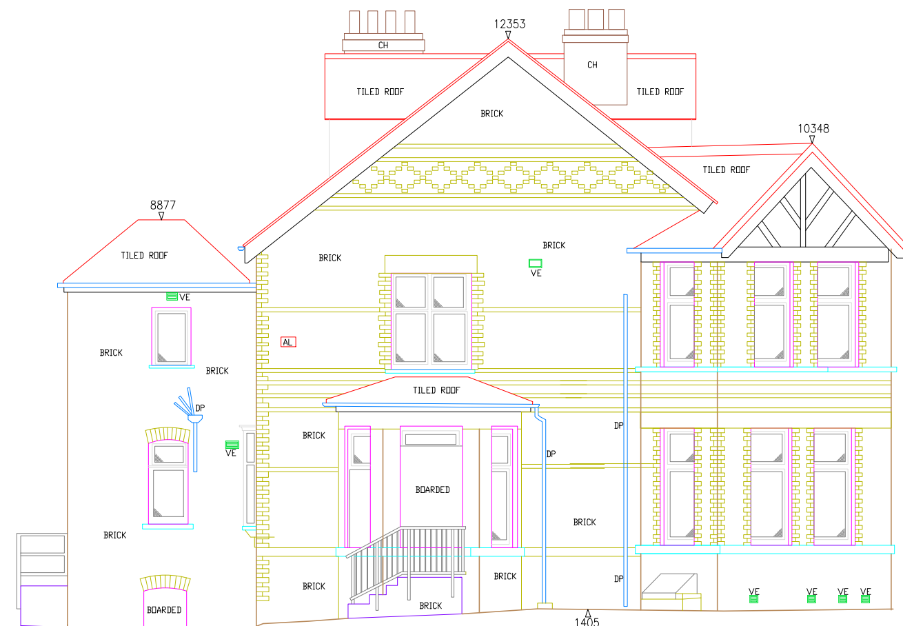
Datum OM EAST ELEVATION
