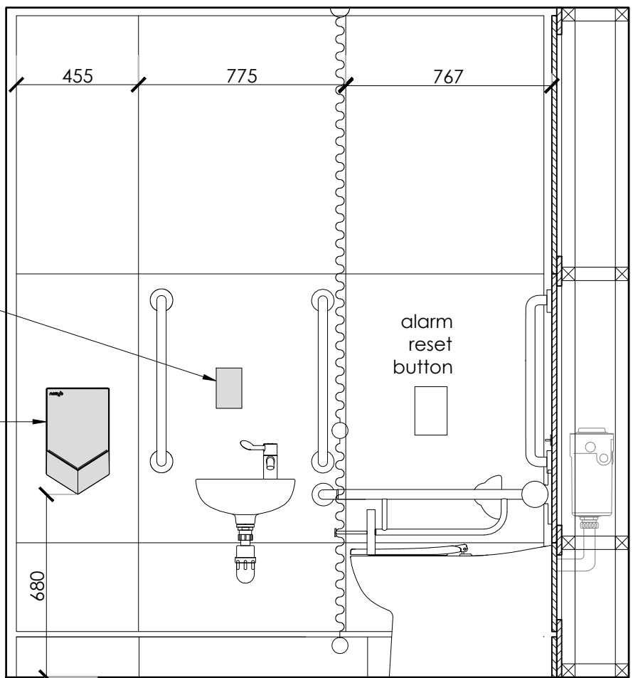
ELEVATION B
