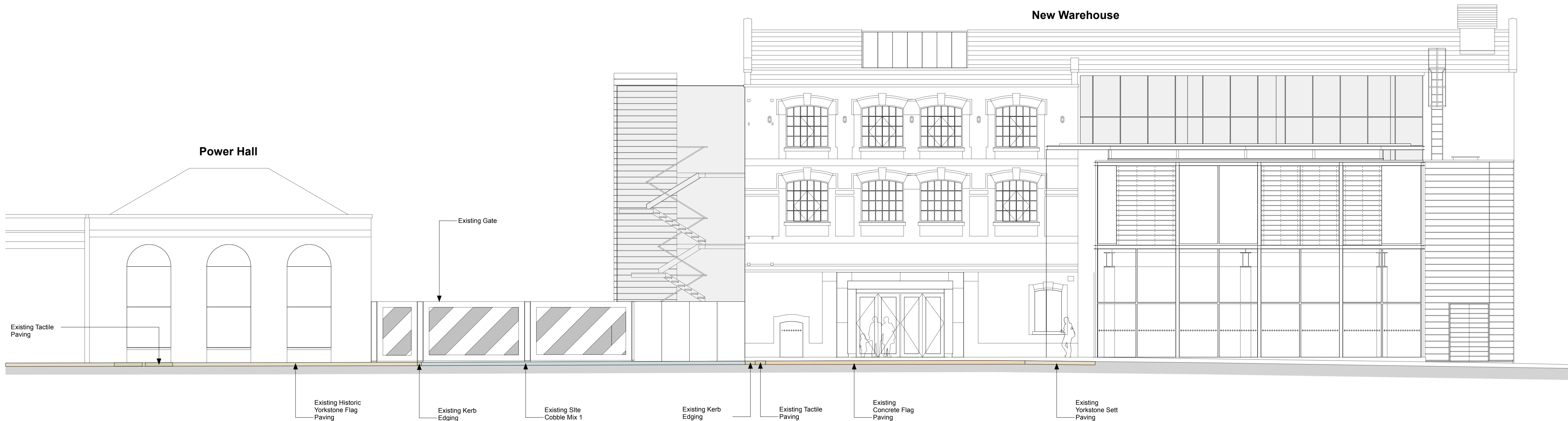
1 Existing Section Elevation A-A Scale: 1:100
