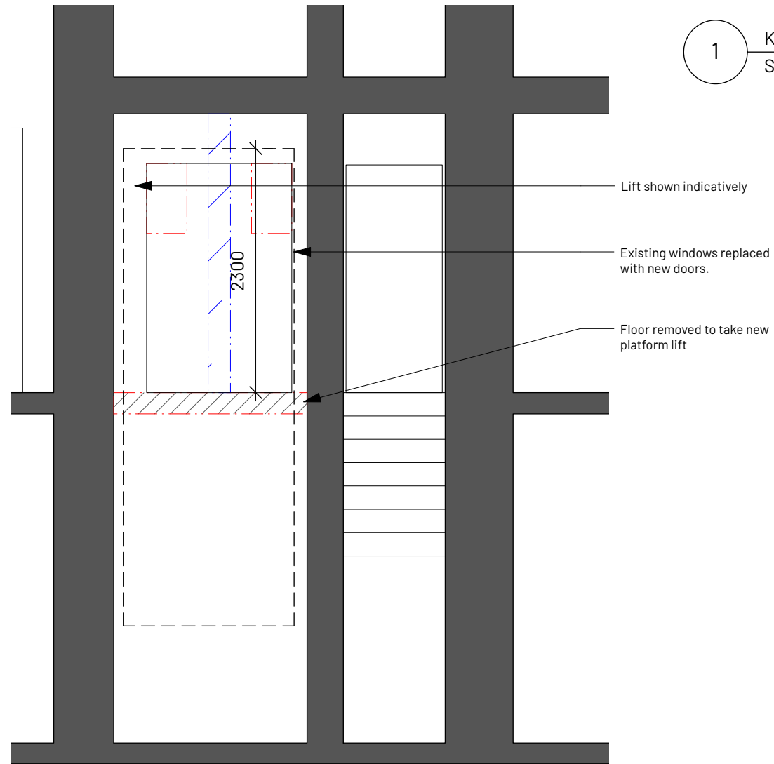
3 Section FF Scale: 1:50
