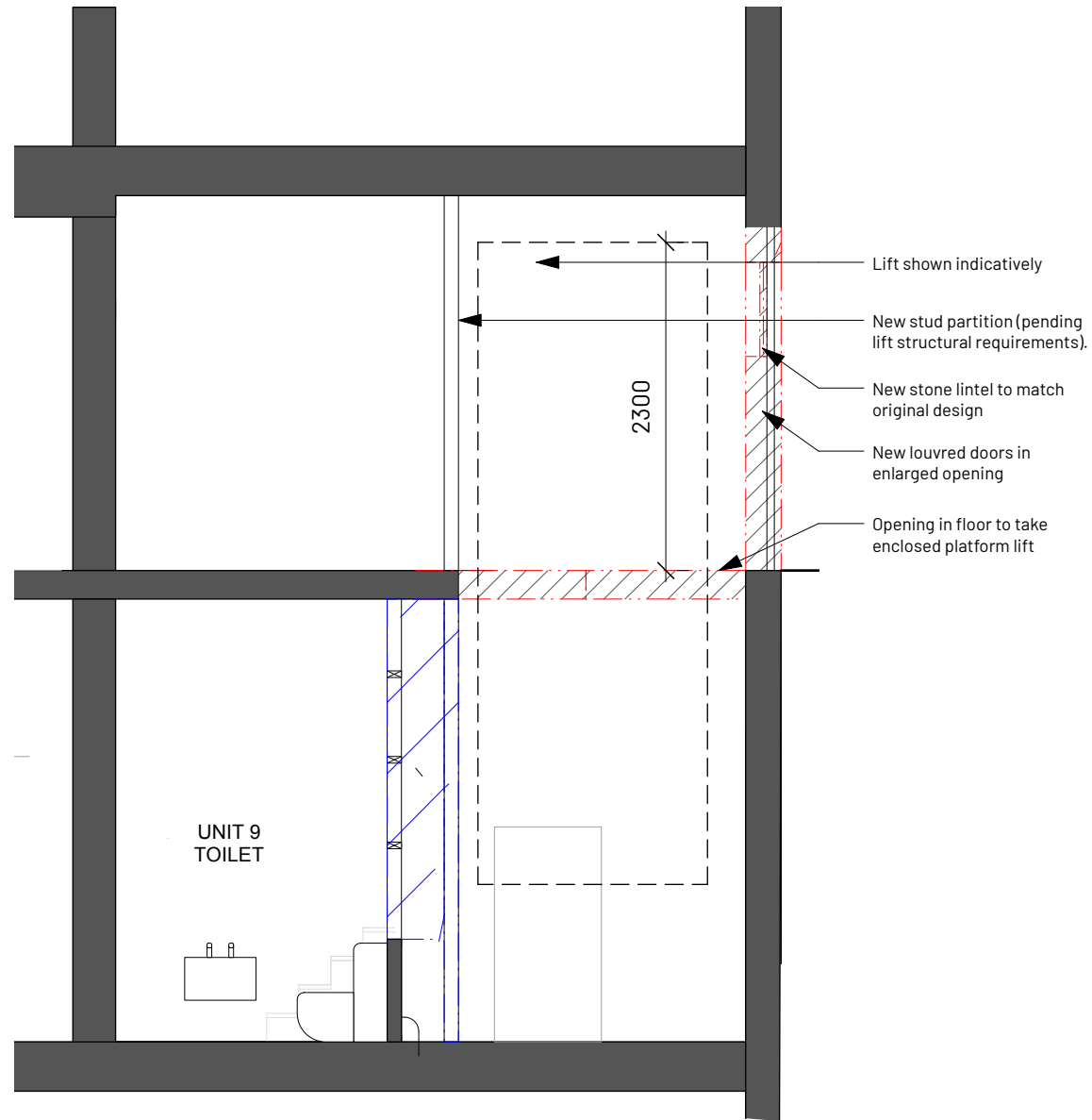
2 Section EE Scale: 1:50
