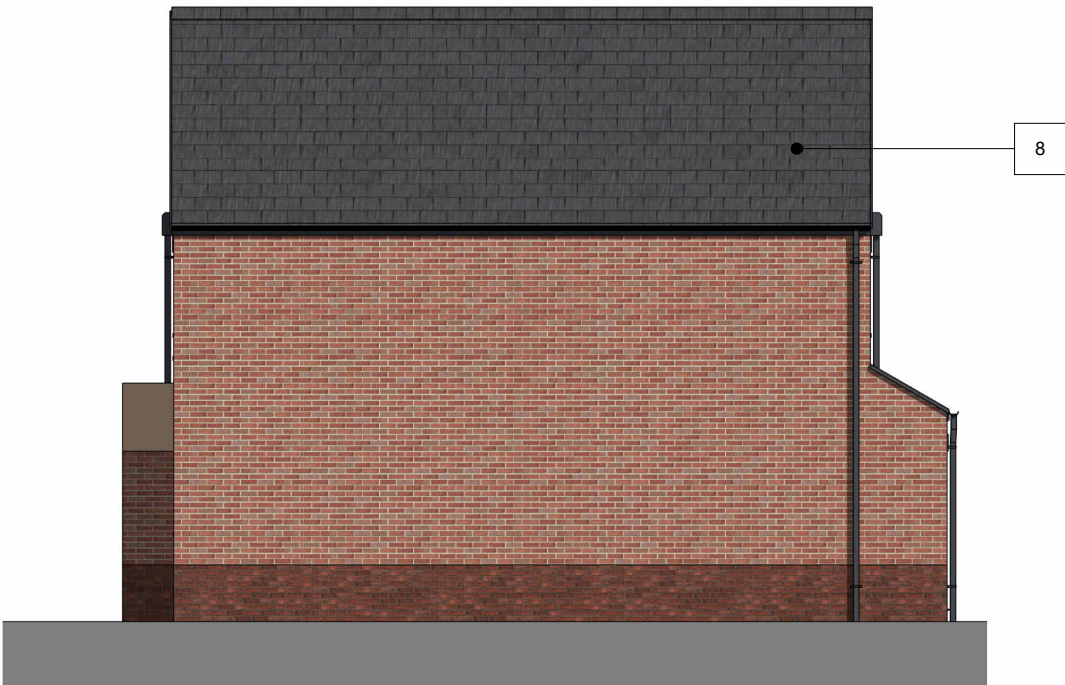
Right Elevation 1 : 100
