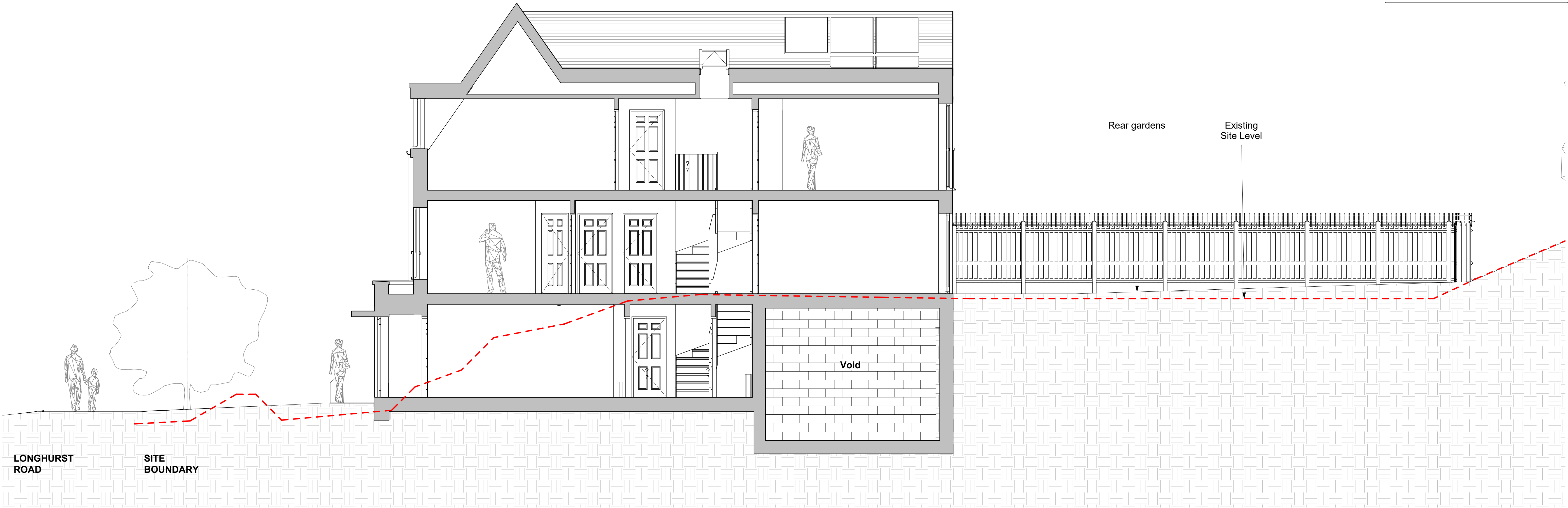
Section 4 - Block 4 1 : 50
