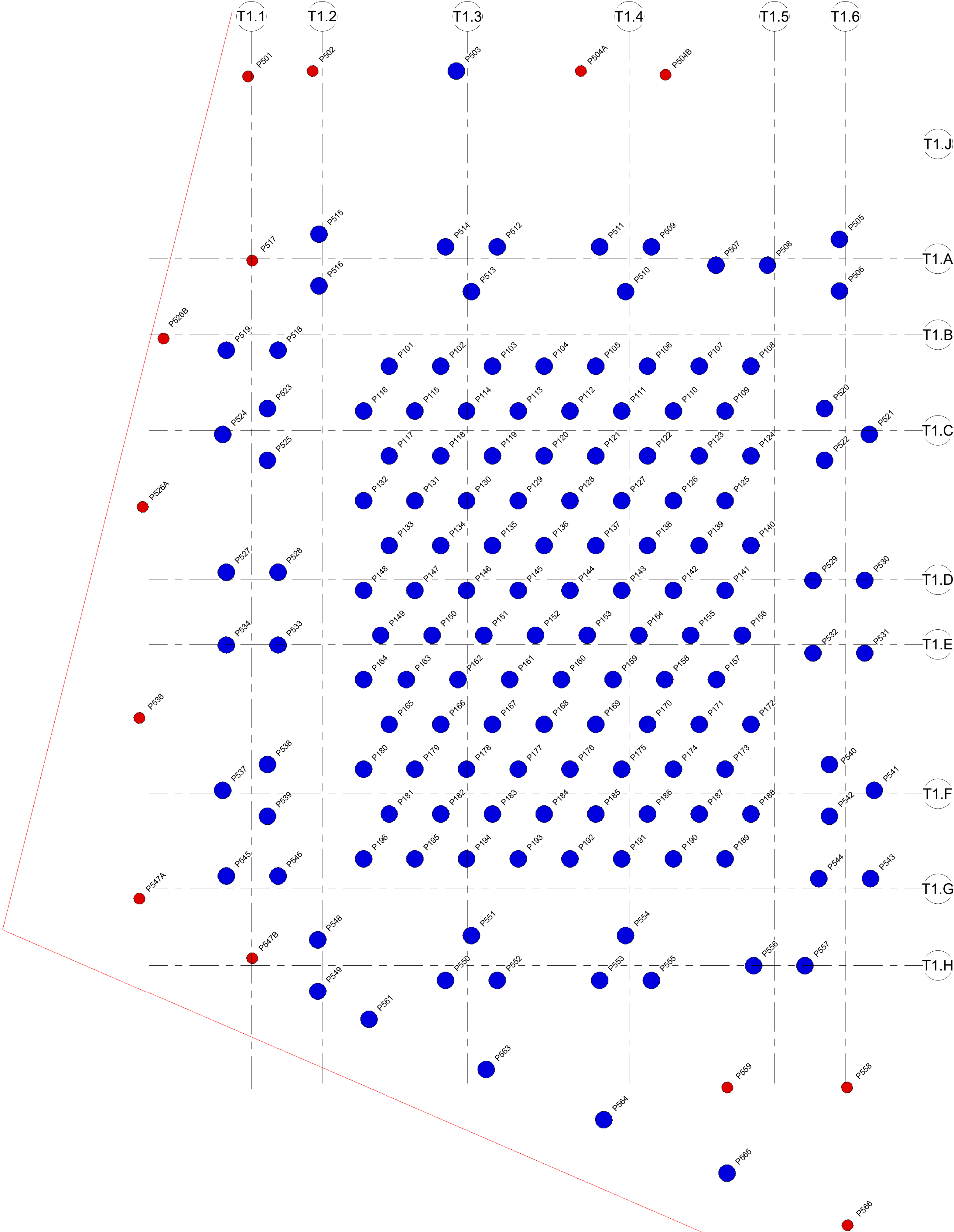
1 PILING PLAN 1 : 100
