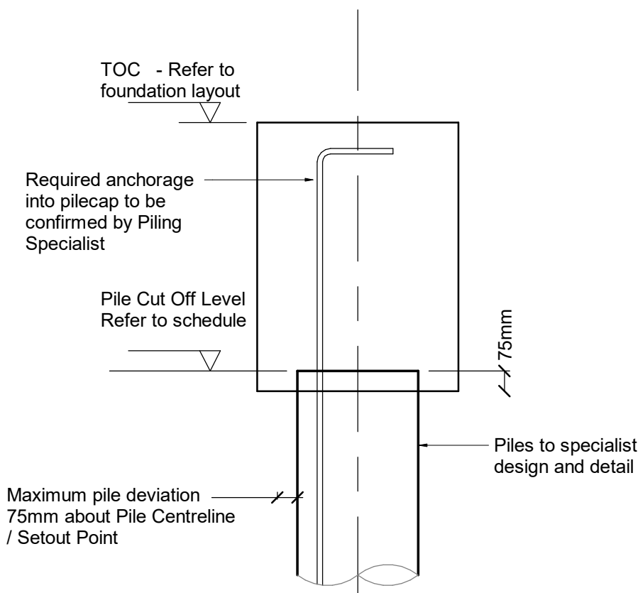
2 PILE DIAGRAM 1 : 20
