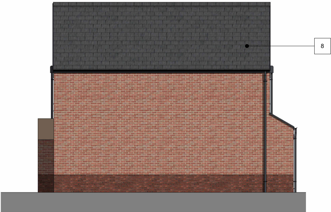
Right Elevation 1 : 100
