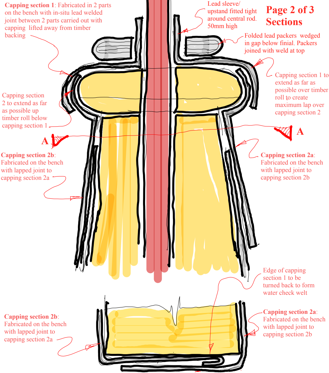
Section A-A
