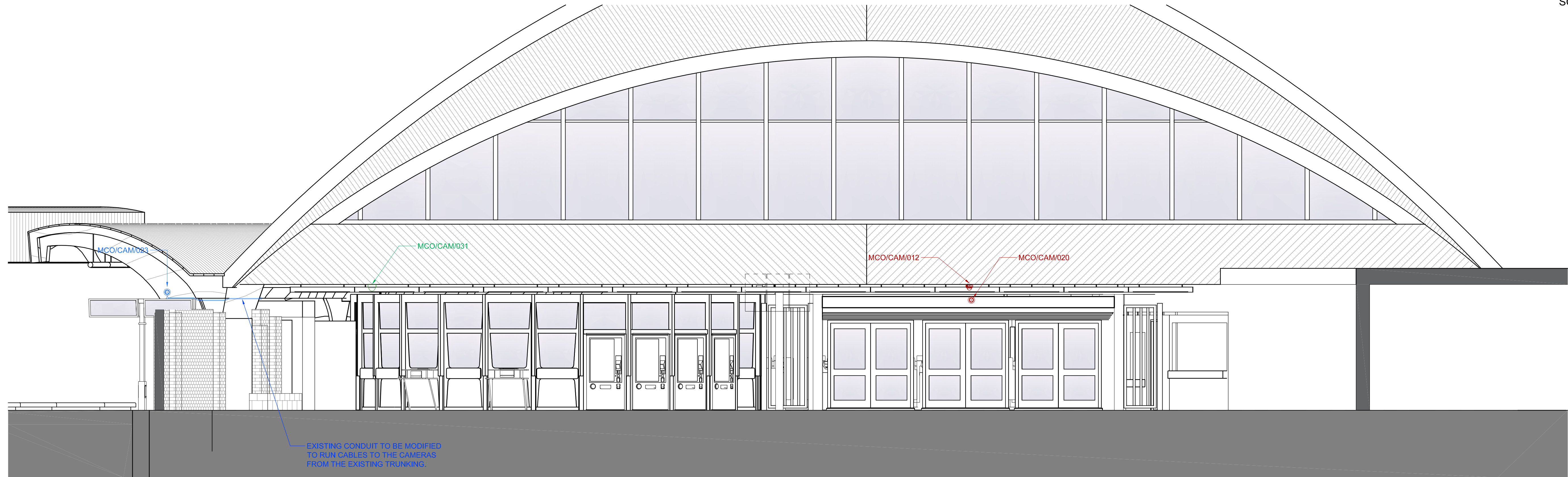
1 SECTION A-A 30 1:50
