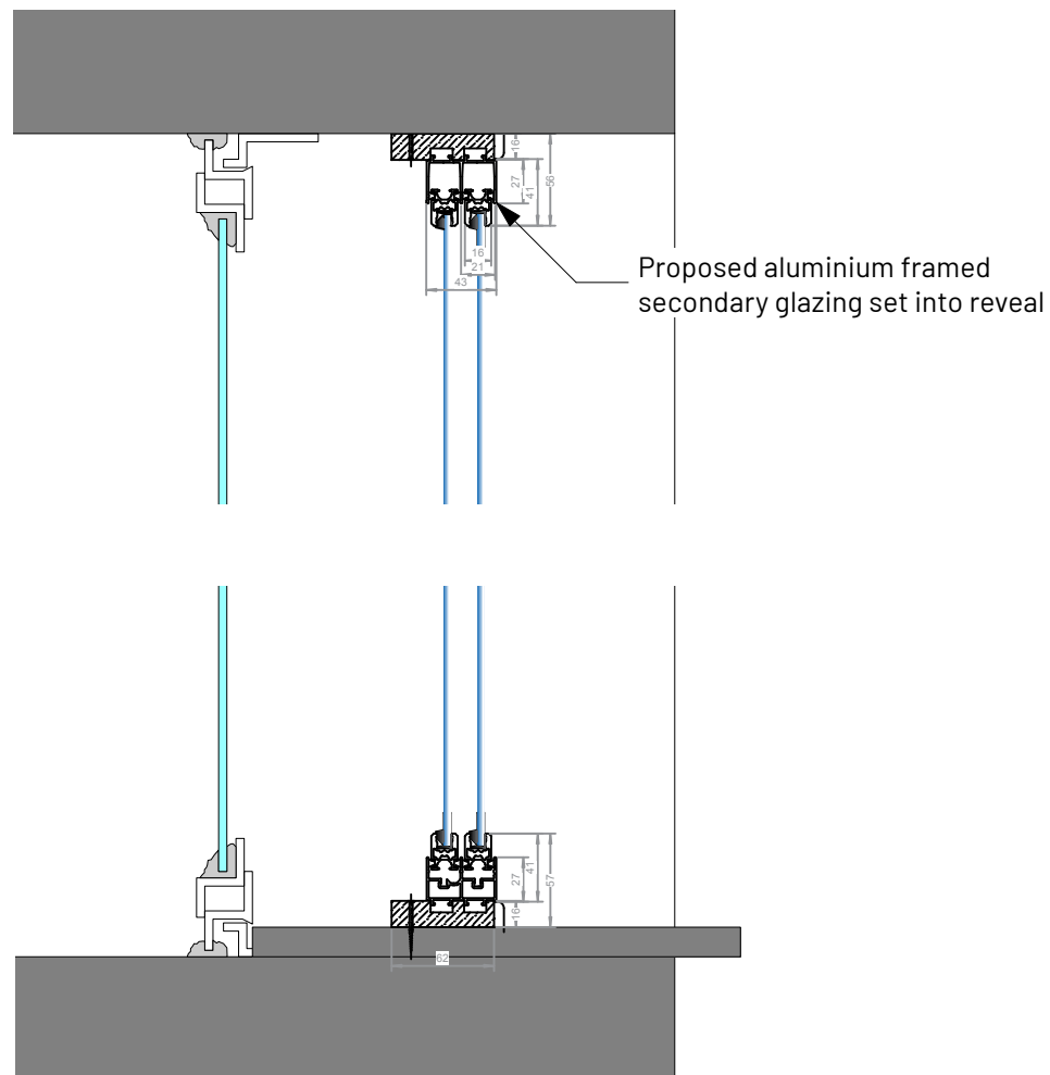
3 Window A Section Scale: 1:5
