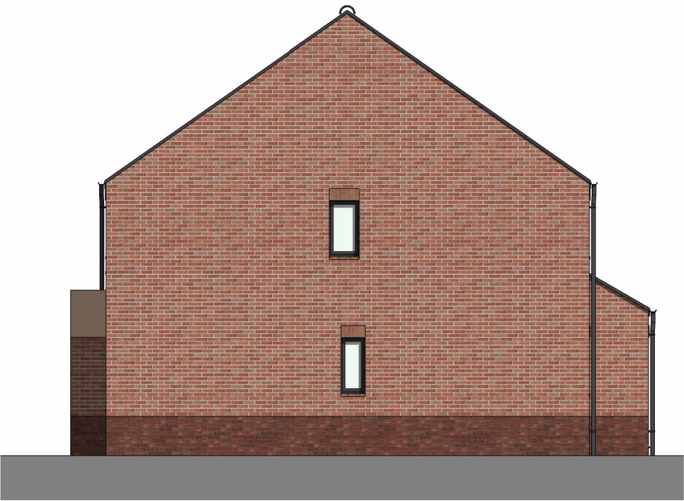
Right Elevation 1 : 100
