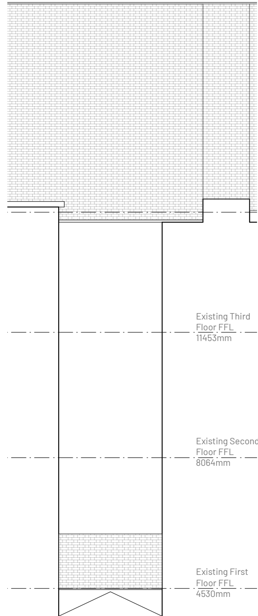
3 Lightwell Elevation BB Scale: 1:100
