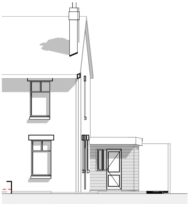
PROP NORTH EL 1:100
