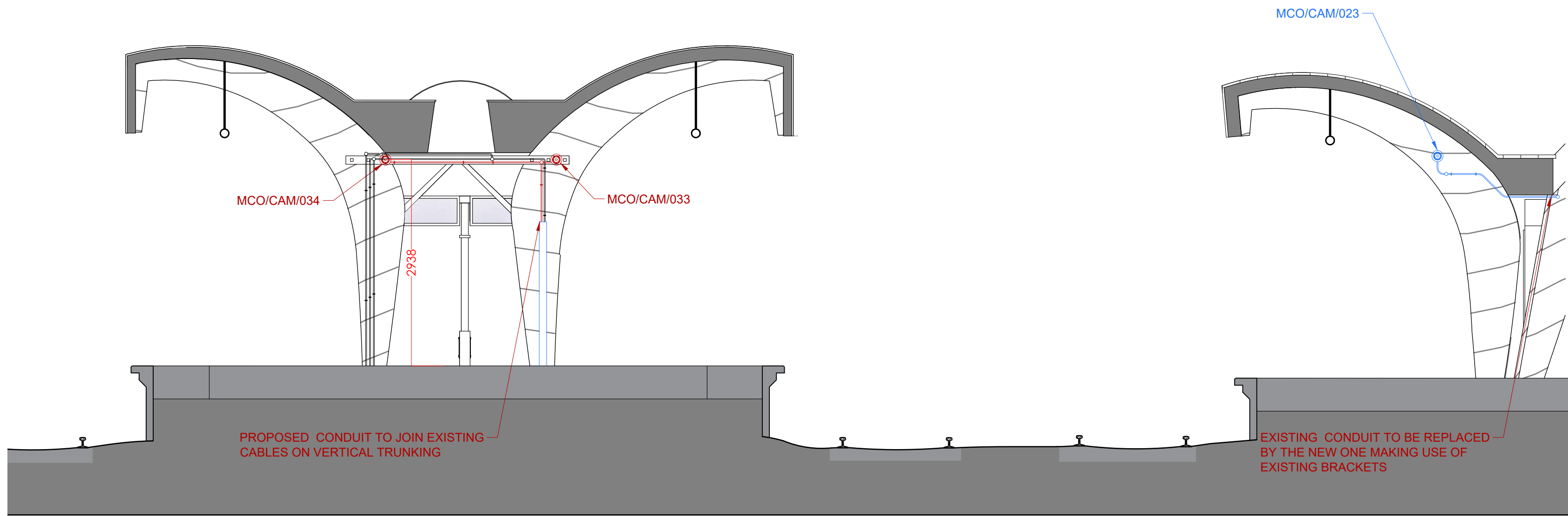
2 SECTION D-D 31 1:50
