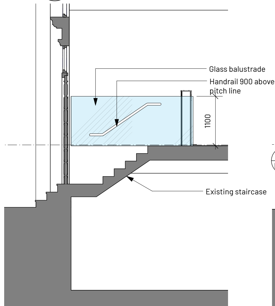
Section AA Scale: 1:50
