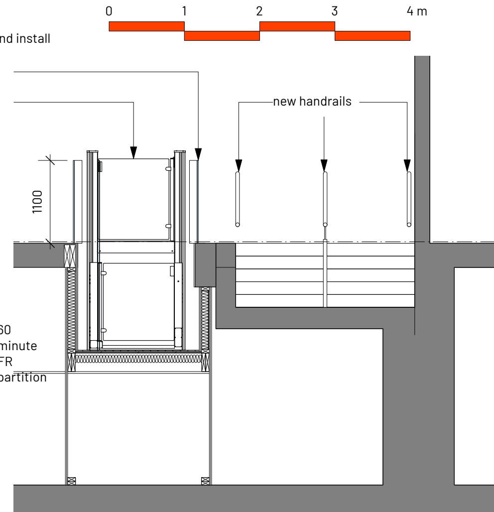
Section CC Scale: 1:50
