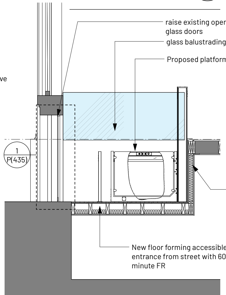
Section BB Scale: 1:50
