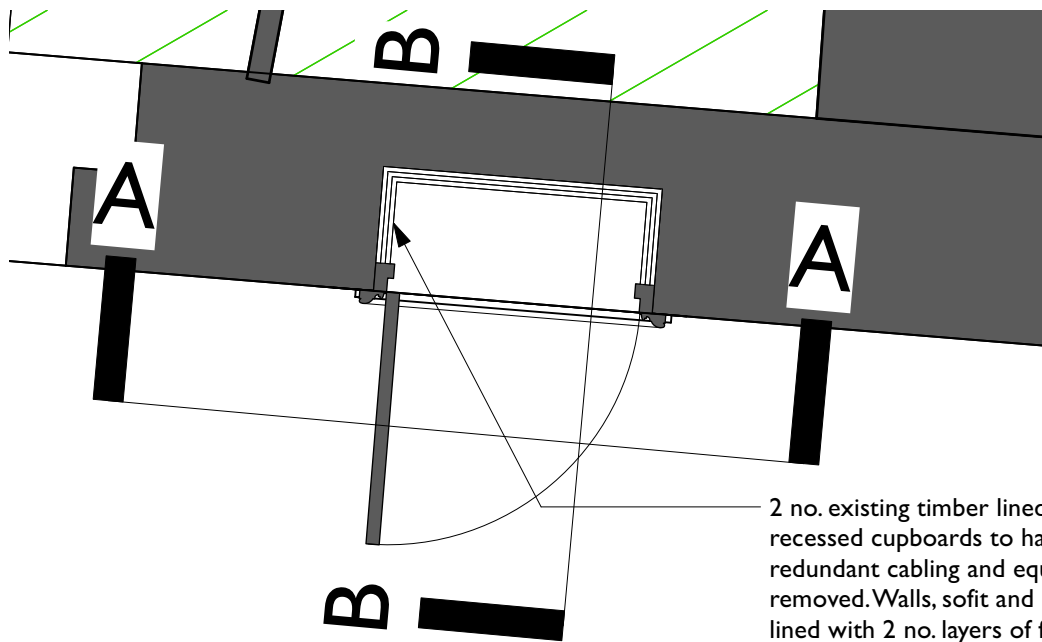
2 Pin 003 I:38 Scale: 1:20
