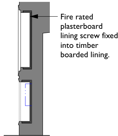
5 Section BB Scale: 1:50
