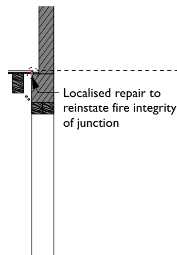
7 Section BB Scale: 1:50
