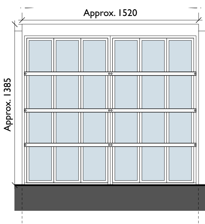
Existing Elevation Scale: 1:20
