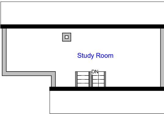
4 Loft Plan 1 : 150
