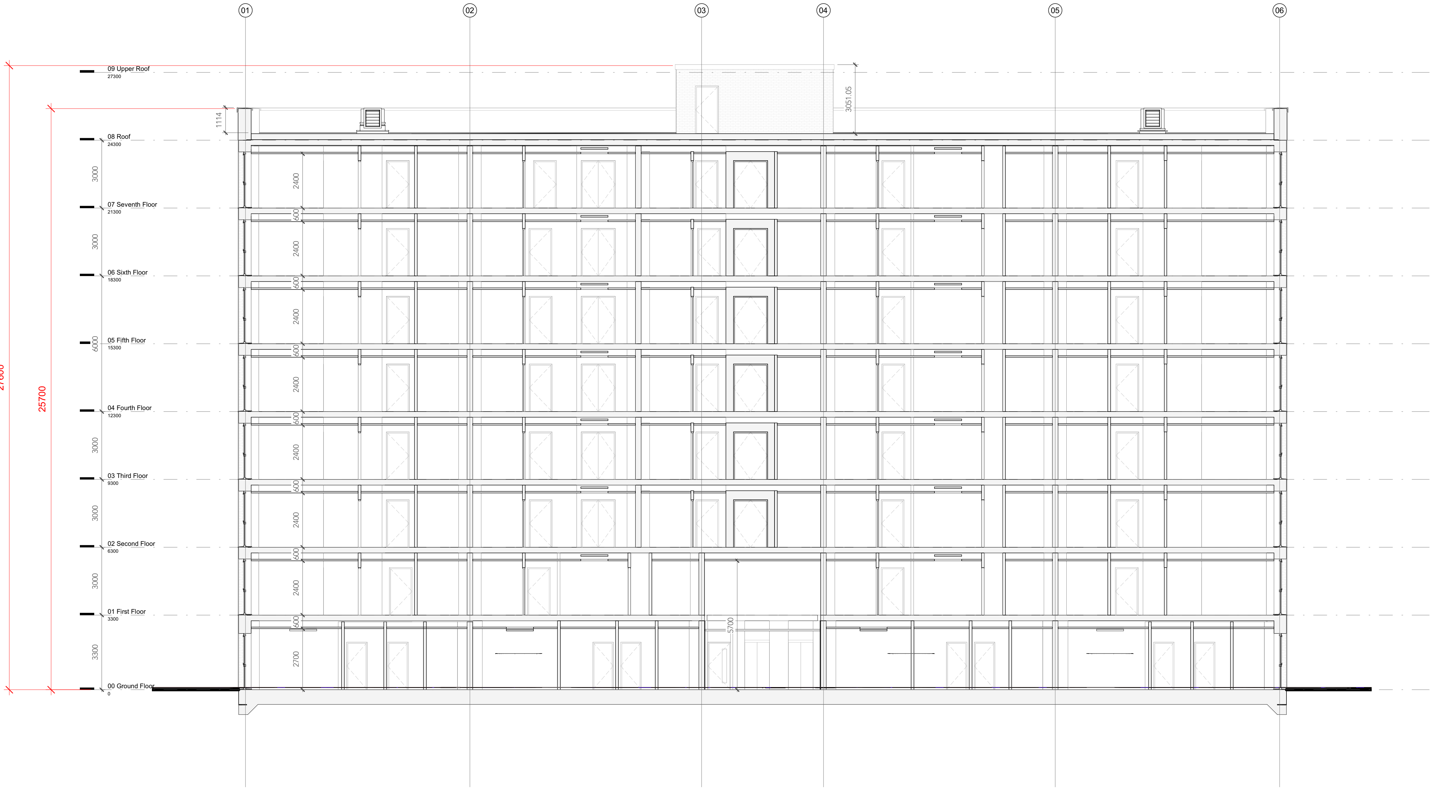
Section AA 1 : 100
