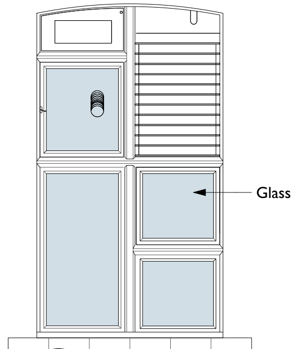
1 Existing Window Elevation Scale: 1:30
