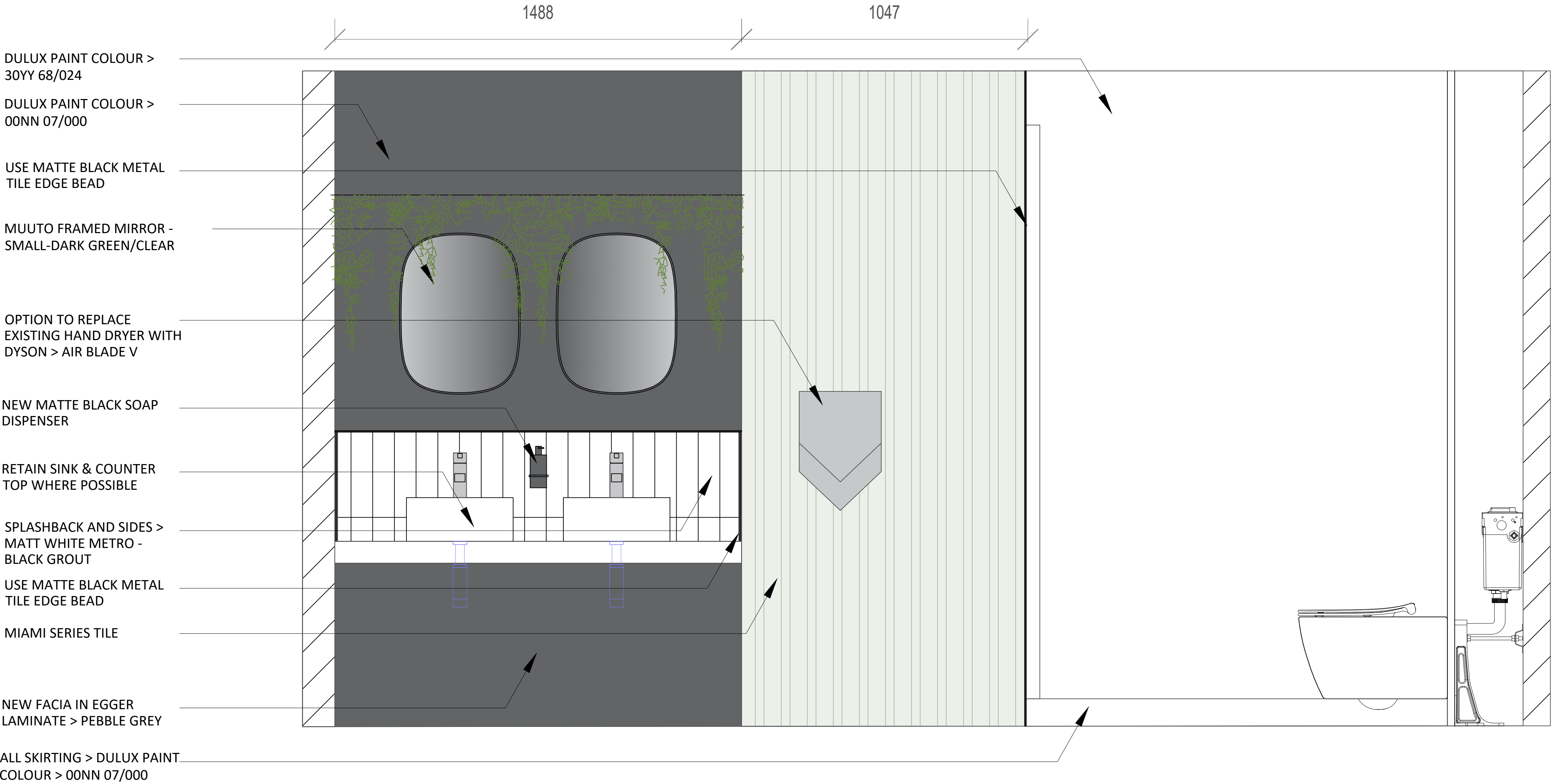
ELEVATION A
