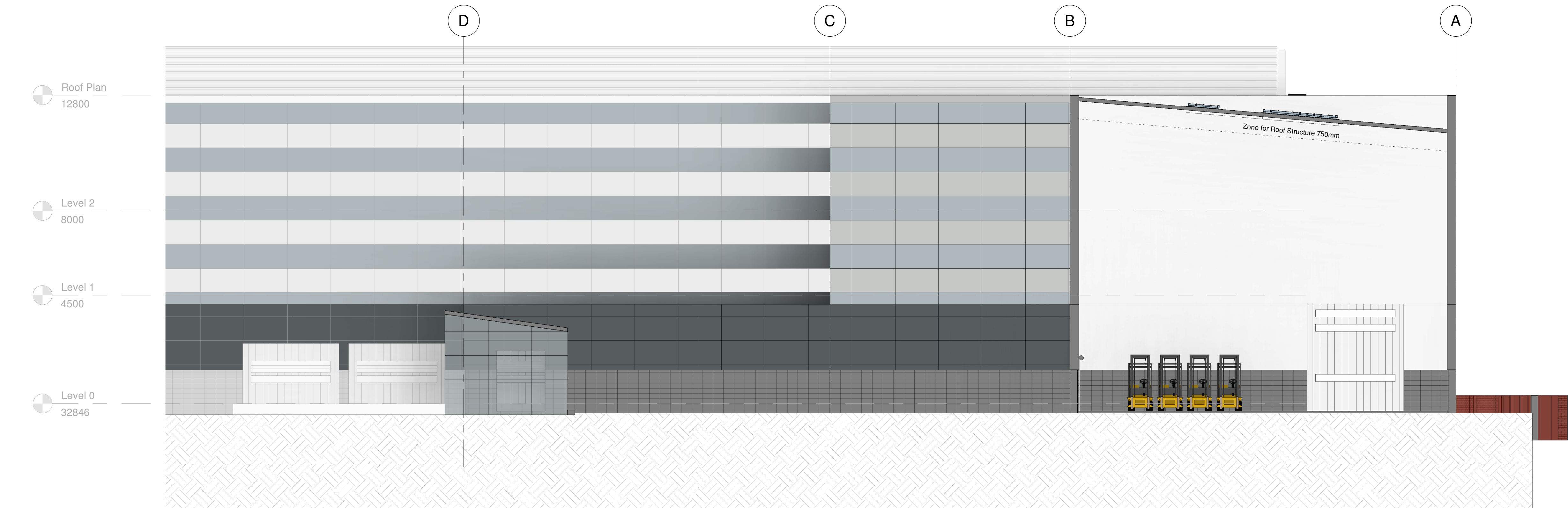
2 Section B 1 : 100
