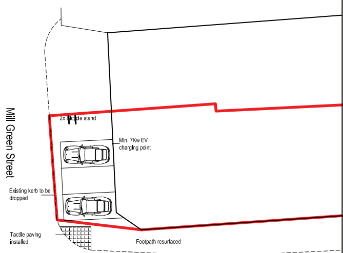
Dark Lane SITE PLAN 1:250
