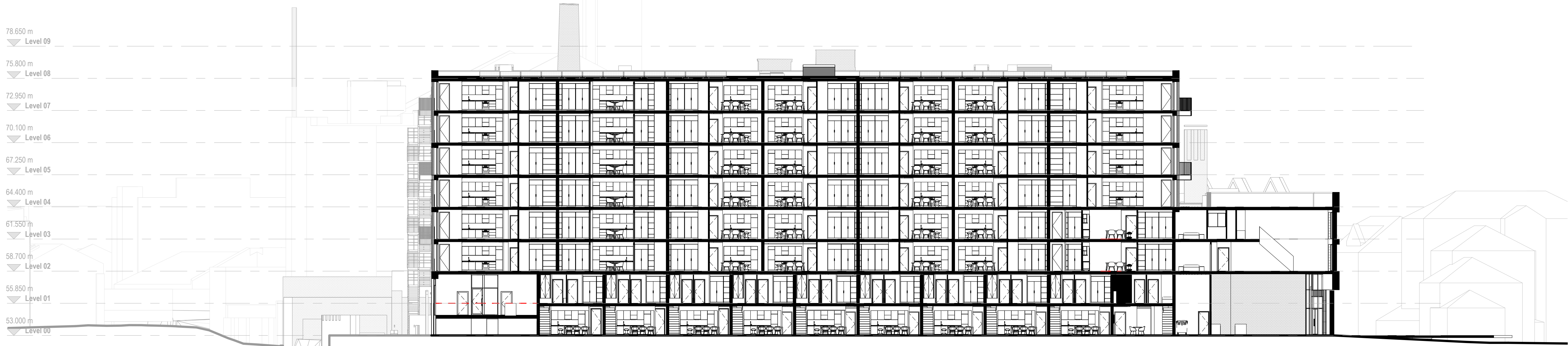
GA Section DD 1 : 200
