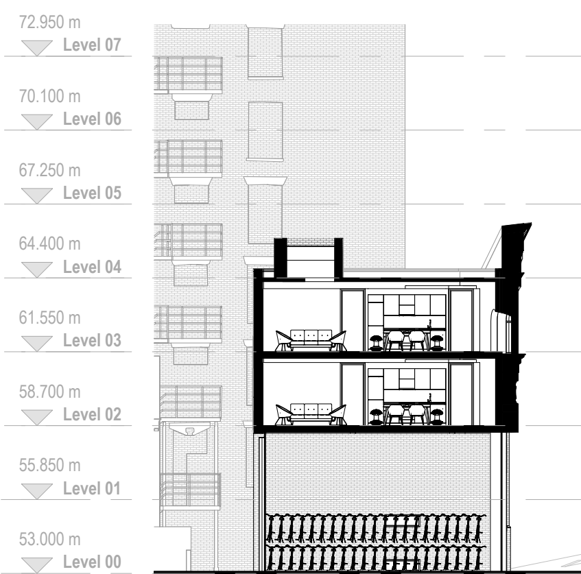
GA Section FF 1 : 200
