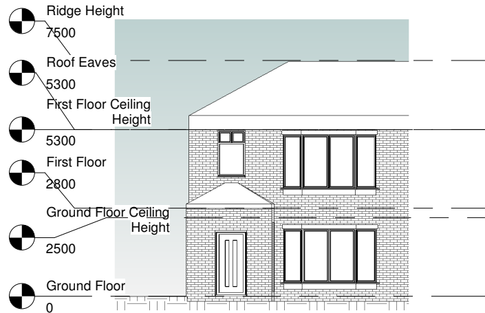
1 North 1 : 100
