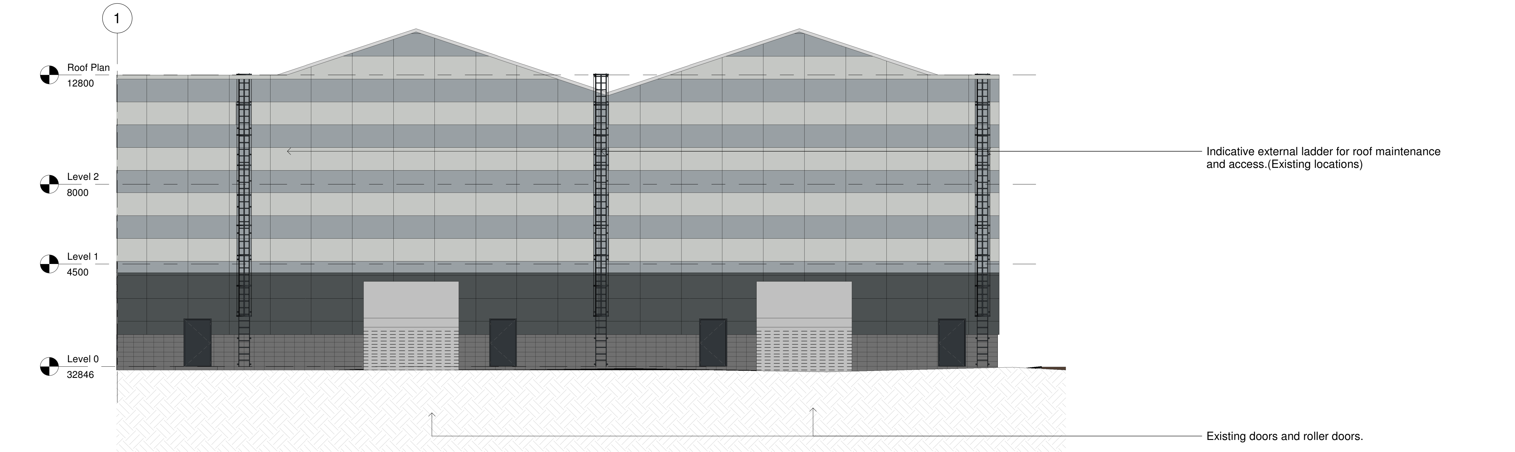
5 Elevation 5 1 : 100
