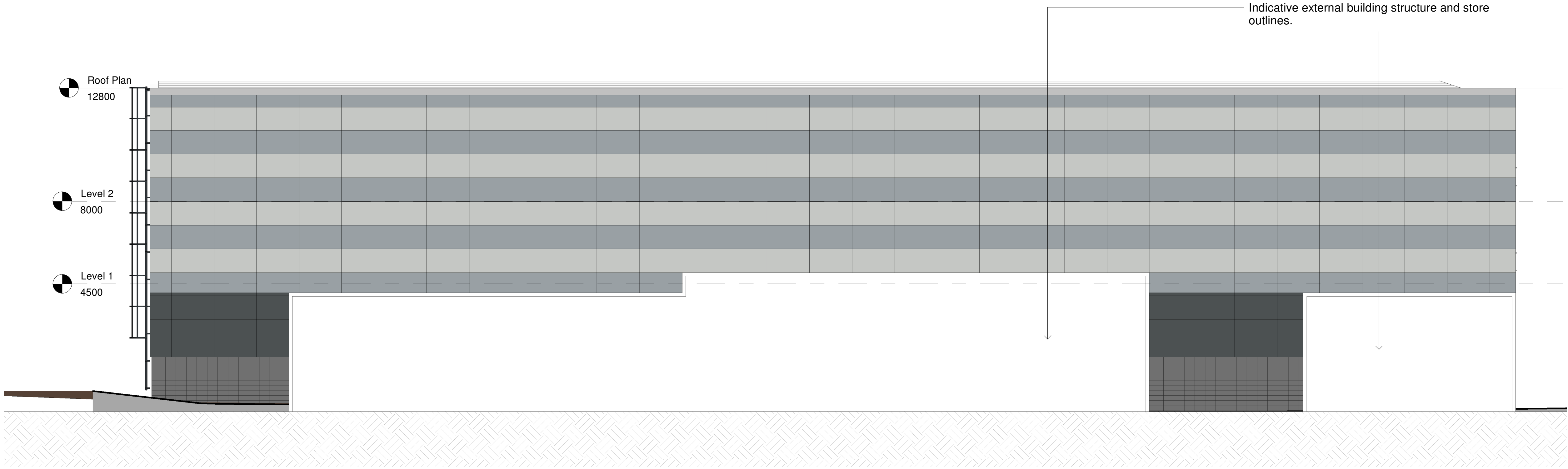
6 Elevation 6 1 : 100
