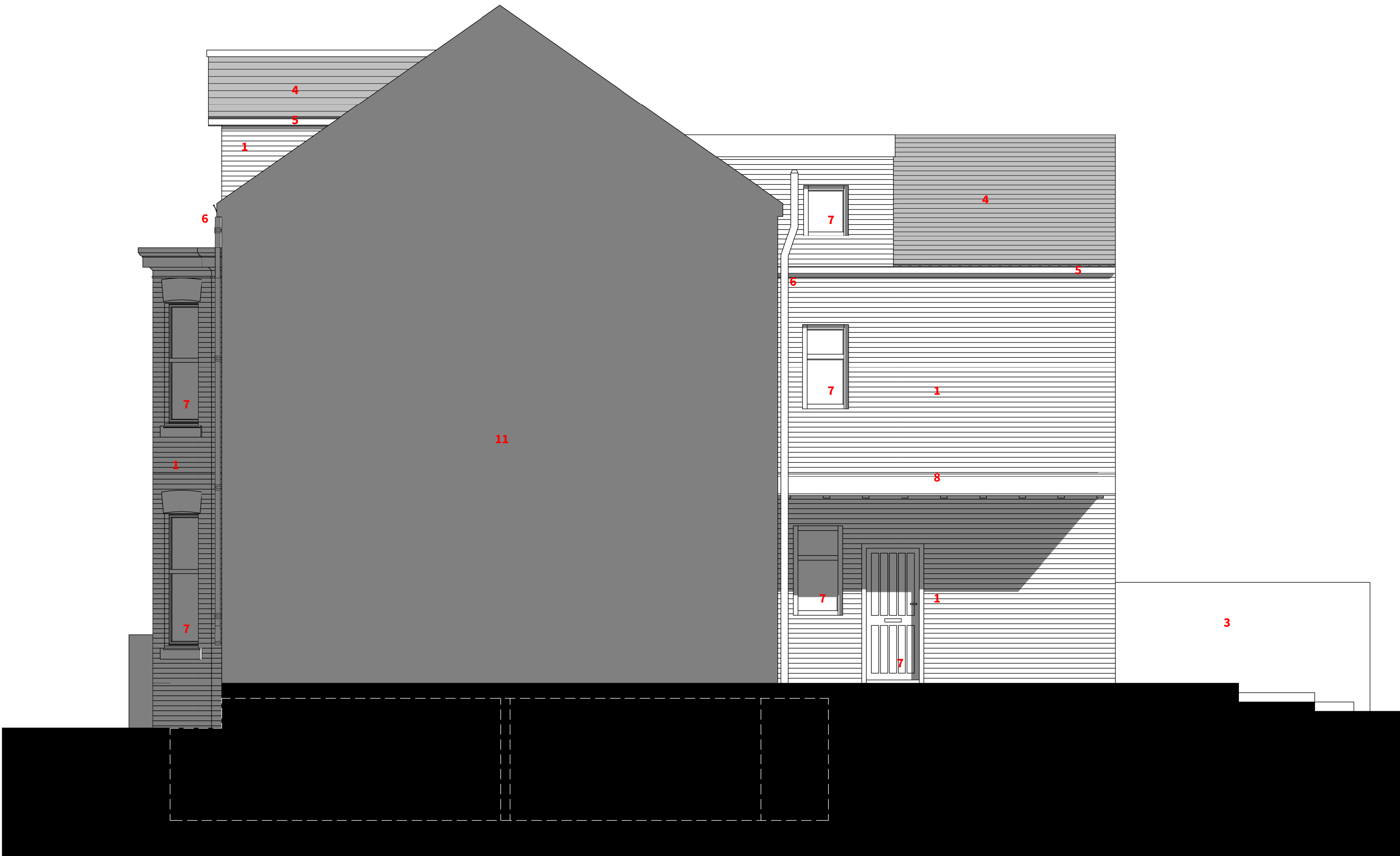
Existing Side Elevation 1:50 / A1 (1:100 / A3)
