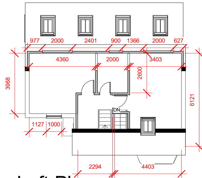
3 Loft Plan 1 : 150
