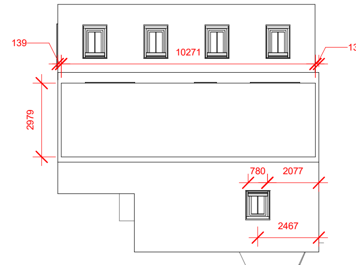
4 Roof Plan 1 : 150
