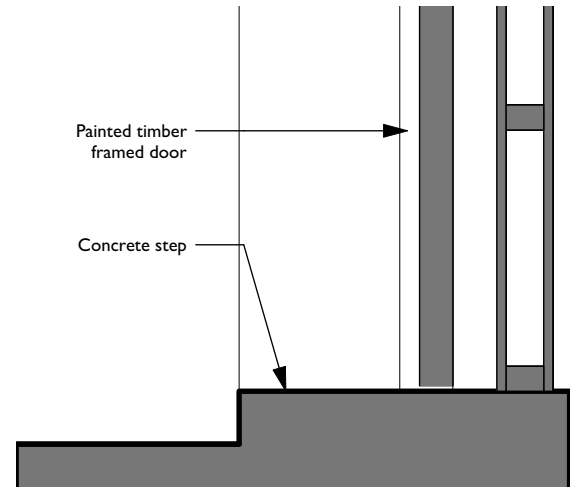
2 Existing Cill Detail Scale: 1:10
