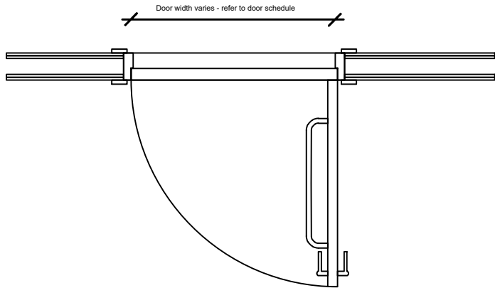
3 Type A3 : Plan 1:25 @ A3
