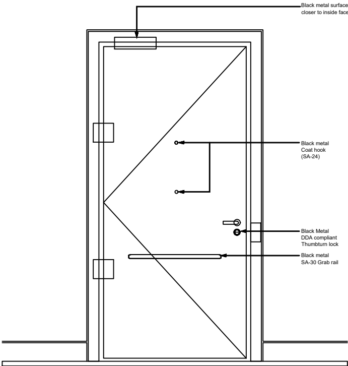
2 Type A3 : Rear Elevation 1:25 @ A3
