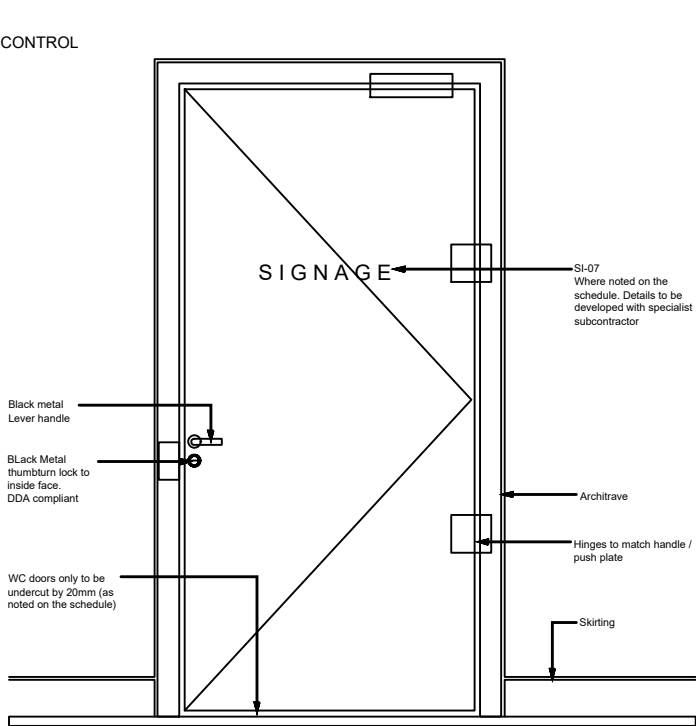
1 Type A3 : Front Elevation 1:25 @ A3
