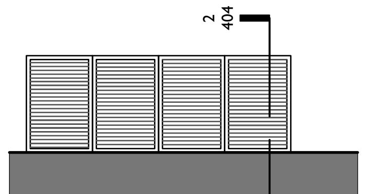
1 Existing Elevation Scale: 1:20
