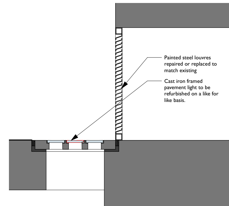
5 Existing Section Scale: 1:10
