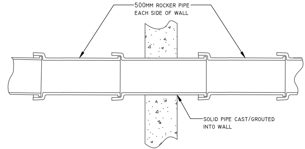
ROCKER PIPE DETAIL N.T.S
