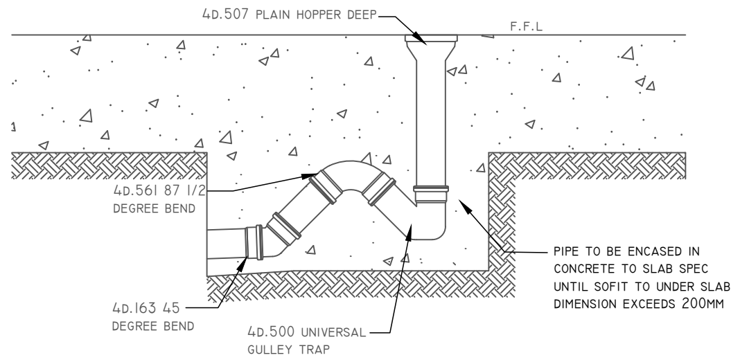
FLOOR GULLY DETAIL N.T.S
