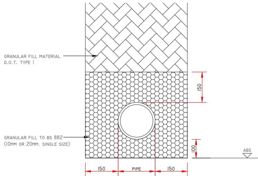
CLASS S PIPE BEDDING N.T.S
