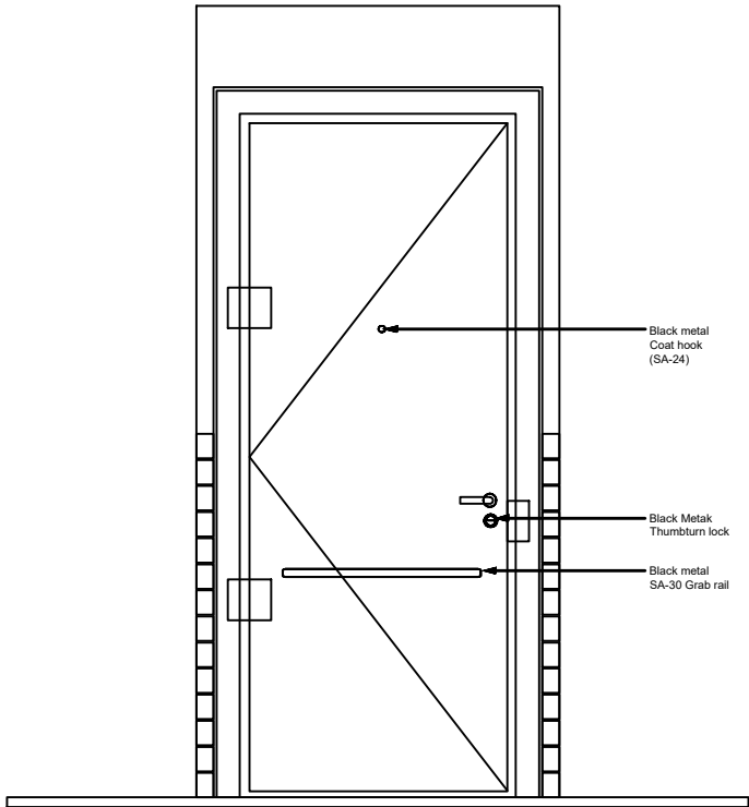
2 Type A2 : Rear Elevation 1:25 @ A3
