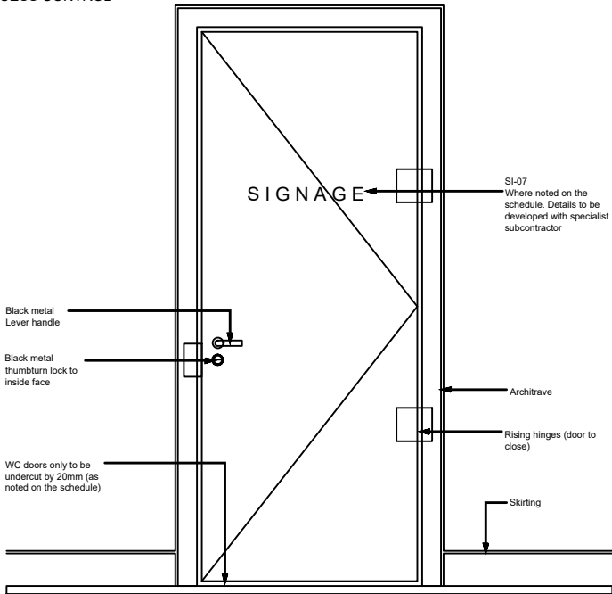
1 Type A2 : Front Elevation 1:25 @ A3
