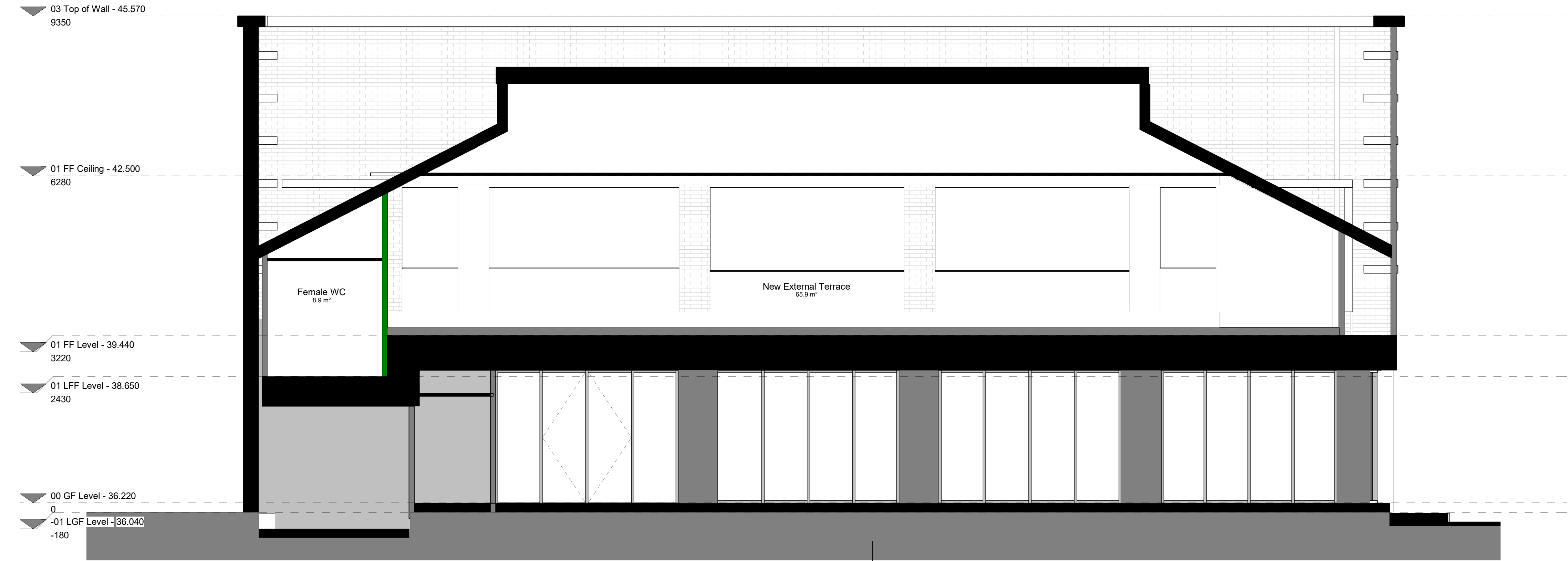
Section BB 1 : 50
