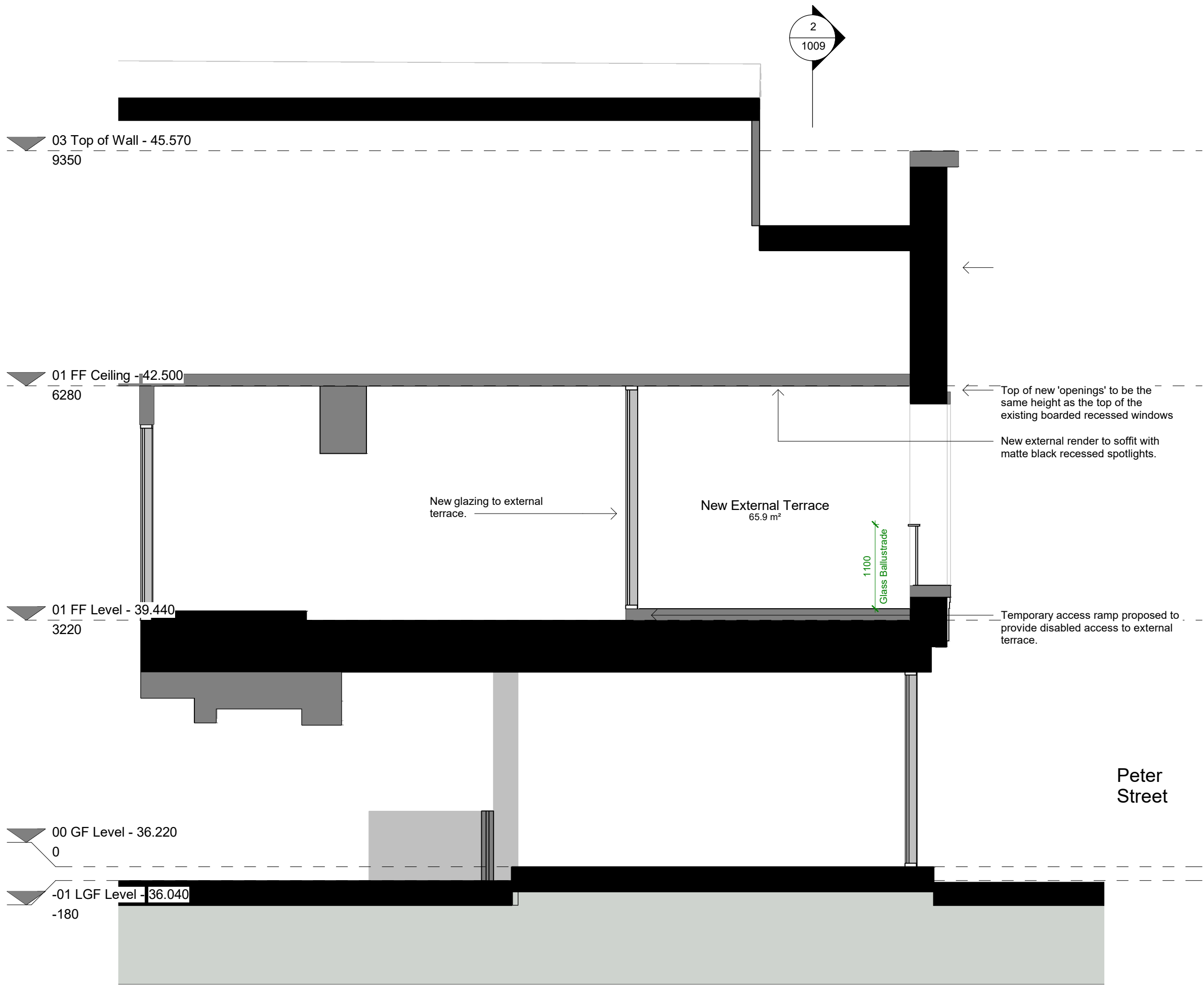
Section AA 1 : 50
